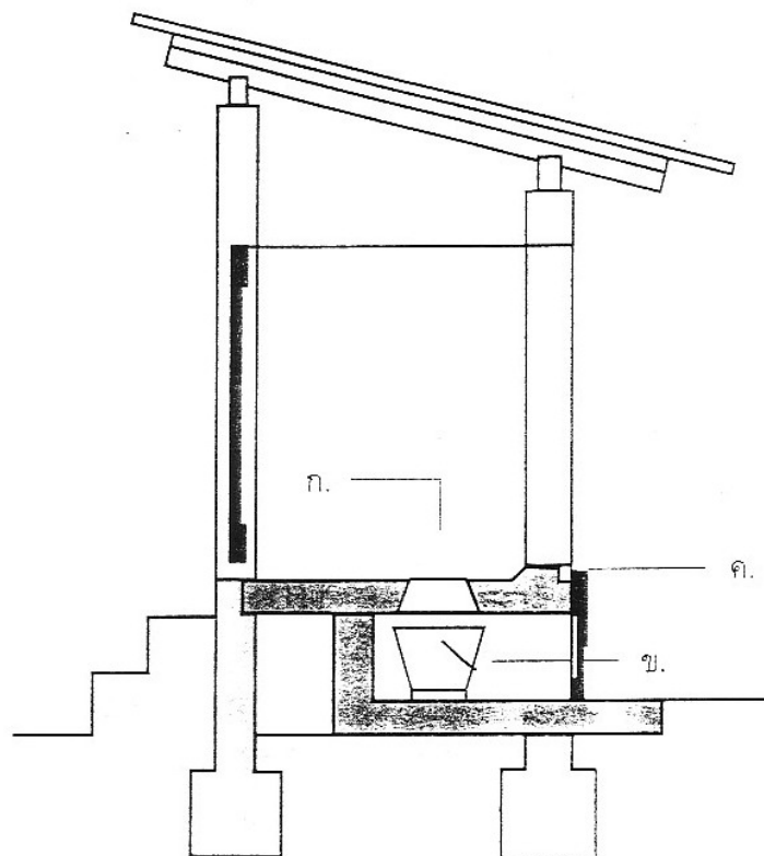
ก. ช่องถ่ายอุจจาระ ข. ถังใส่อุจจาระ ค. แผ่นปิดกันแมลง
