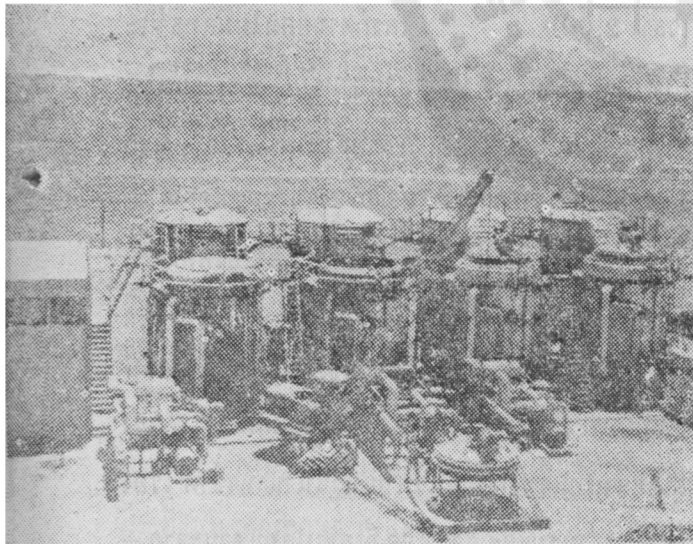
โรงกลั่นน้ำทะเลให้เป็นน้ำดื่มในเมืองท่าอิลลาธ
