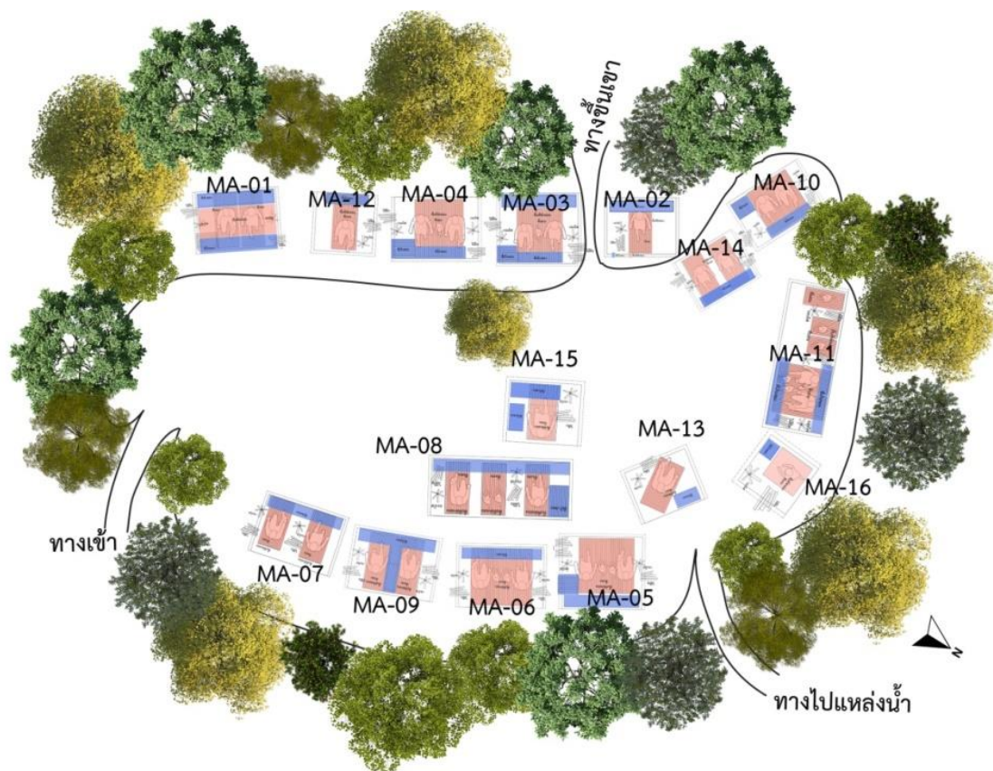
ภาพประกอบ 22 ผังบริเวณการตั้งถิ่นฐานวิถีชีวิตเร่ร่อนดั้งเดิม กลุ่มกองหระ บริเวณน้ำตกไพรวัลย์ จากการเข้าภาคสนามครั้งที่ 2 (ภาพเขียนโดยผู้วิจัย)
