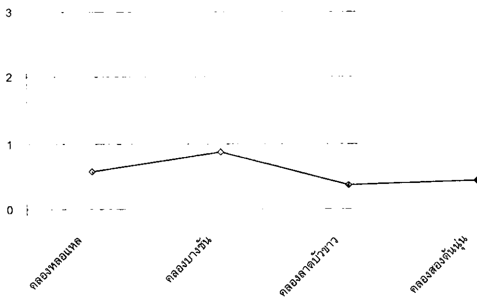
กราฟที่ 53 ปริมาณฟอสฟอรัสทั้งหมดในน้ำคลองย่อย 4 คลอง ในเดือนพฤษภาคม 2544
