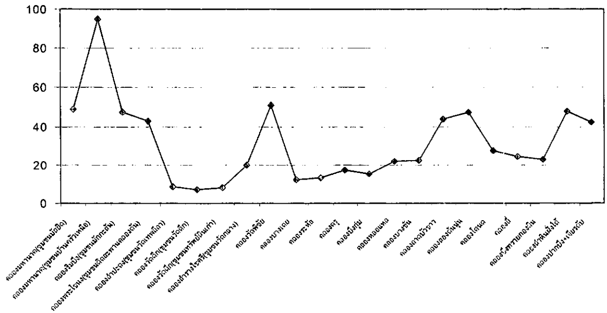
กราฟที่ 61 ปริมาณของแข็งแขวนลอยทั้งหมดในน้ำคลองย่อย 22 คลอง ในเดือนตุลาคม 2544
