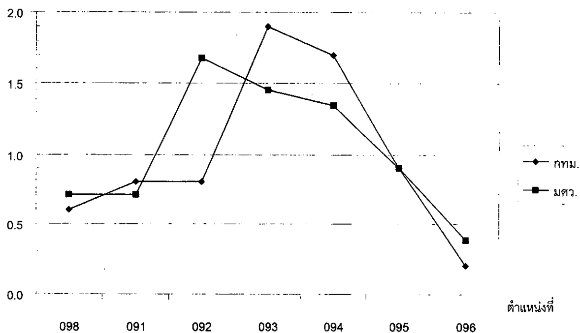
กราฟที่ 35 ปริมาณฟอสฟอรัสทั้งหมดในน้ำคลองแสนแสบในระหว่างเดือนพฤษภาคม - กรกฎาคม 2544
