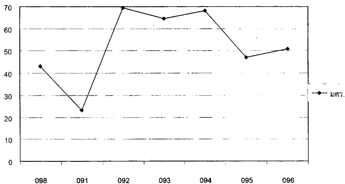
กราฟที่ 11 ปริมาณไนไตรต์ในน้ำคลองแสนแสบในระหว่างเดือนเมษายน - มิถุนายน 2544
