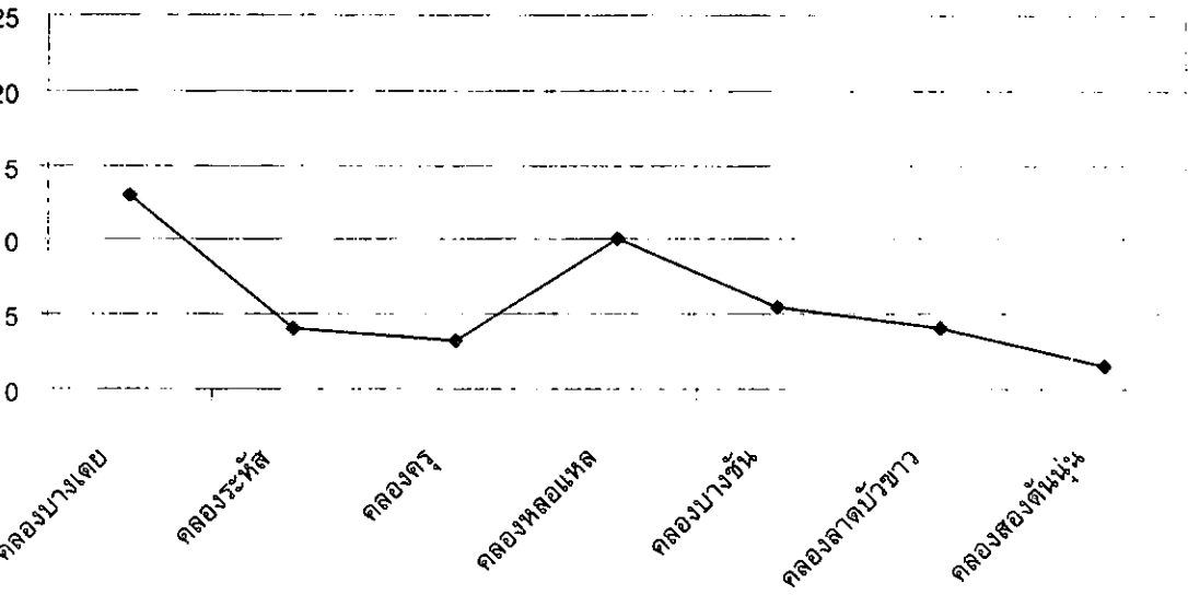
กราฟที่ 40 ปริมาณบีโอดีในน้ำคลองย่อย 7 คลอง ในเดือนกรกฎาคม 2544
