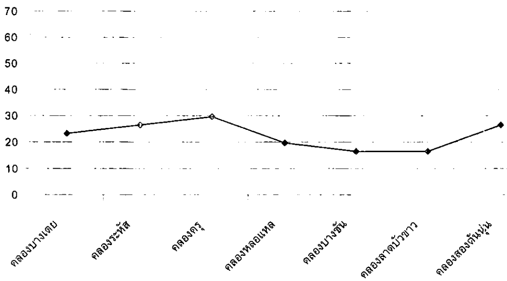
กราฟที่ 42 ปริมาณน้ำดีในน้ำคลองย่อย 7 คลอง ในเดือนกรกฎาคม 2544
