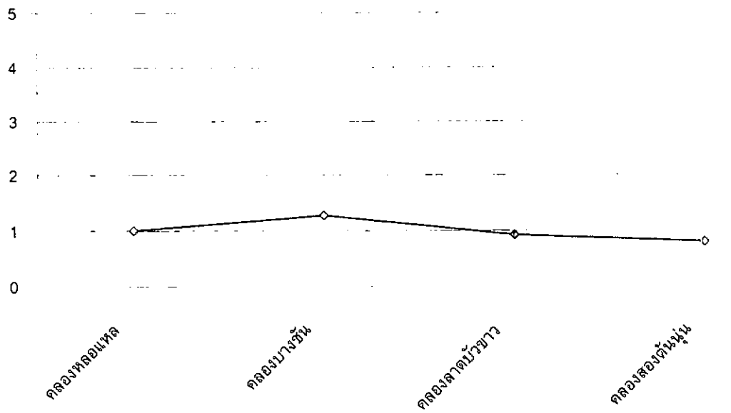
กราฟที่ 37 ปริมาณออกซิเจนละลายในน้ำคลองย่อย 4 คลอง ในเดือนพฤษภาคม 2544
