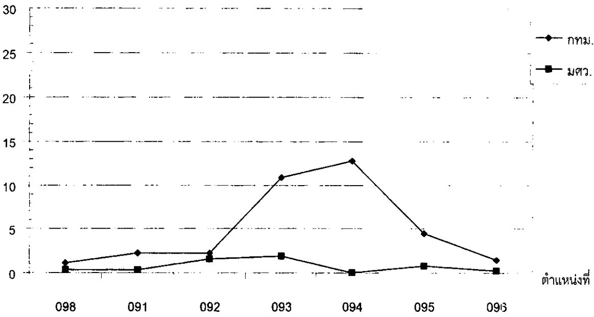
กราฟที่ 27 ปริมาณแอมโมเนียในหน่วยไนโตรเจนในน้ำคลองแสนแสบในระหว่าง เดือนเมษายน - มิถุนายน 2544
