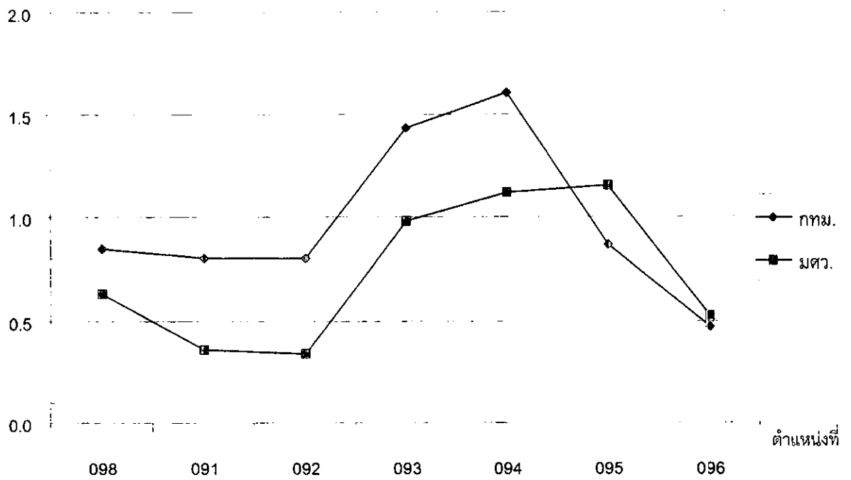
กราฟที่ 34 ปริมาณฟอสฟอรัสทั้งหมดในน้ำคลองแสนแสบในระหว่างเดือนมกราคม - มีนาคม 2544
