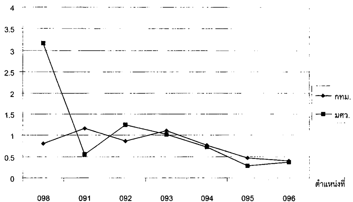
กราฟที่ 36 ปริมาณฟอสฟอรัสทั้งหมดในน้ำคลองแสนแสบในระหว่างเดือนกรกฎาคม -- กันยายน 2544
