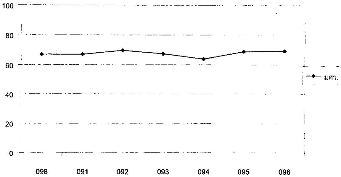
กราฟที่ 19 ปริมาณคลอรีนในน้ำคลองแสนแสบในระหว่างเดือนเมษายน – มิถุนายน 2544
