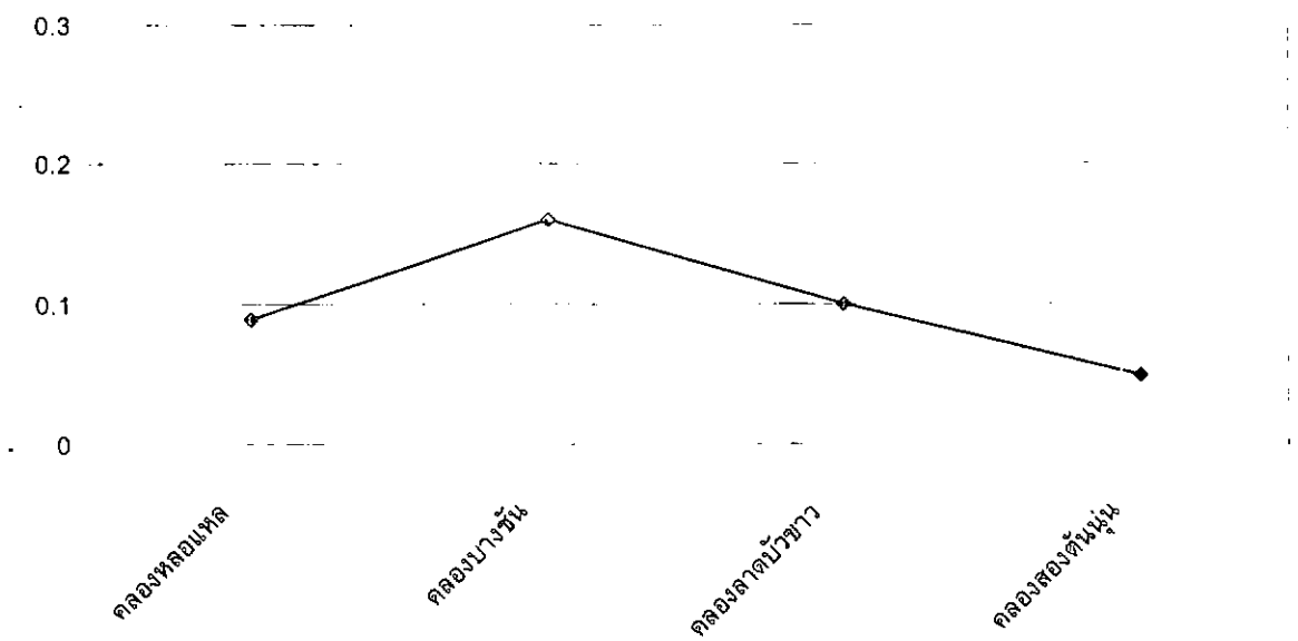
กราฟที่ 49 ปริมาณแอมโมเนียในหน่วยไนโตรเจนในน้ำคลองย่อย 4 คลอง ในเดือนพฤษภาคม 2544
