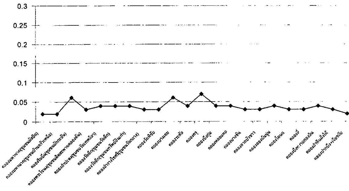
กราฟที่ 68 ปริมาณแอมโมเนียในหน่วยไนโตรเจนในน้ำคลองย่อย 22 คลอง ในเดือนพฤศจิกายน 2544
