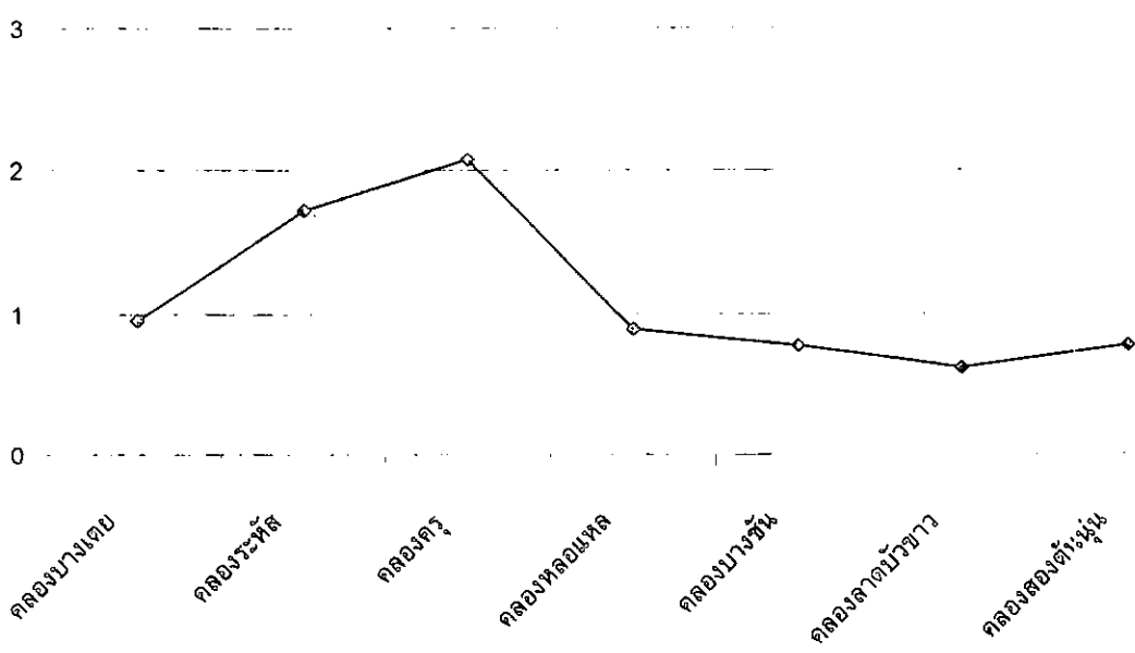
กราฟที่ 54 ปริมาณฟอสฟอรัสทั้งหมดในน้ำคลองย่อย 7 คลอง ในเดือนกรกฎาคม 2544
