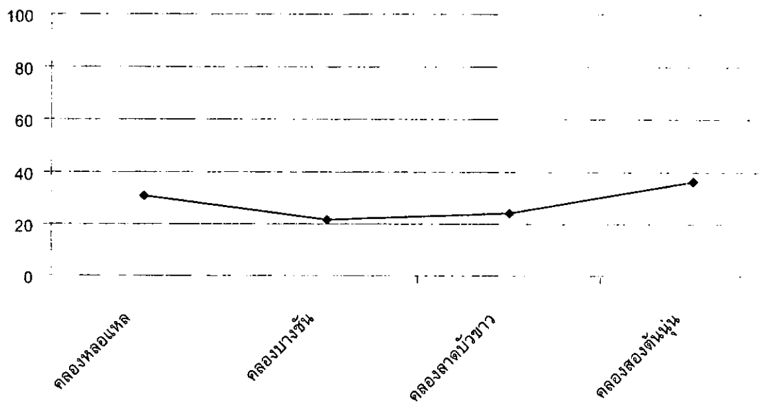
กราฟที่ 43 ปริมาณของแข็งแขวนลอยทั้งหมดในน้ำคลองย่อย 4 คลอง ในเดือนพฤษภาคม 2544
