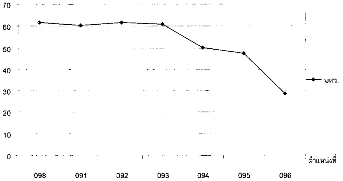
กราฟที่ 9 ปริมาณซีไอดีในน้ำคลองแสนแสบในเดือนธันวาคม 2543
