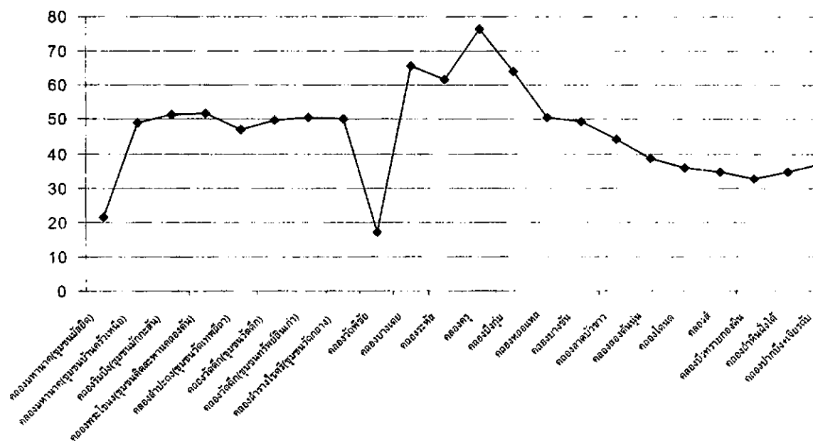
กราฟที่ 63 ปริมาณคลอไรด์ในน้ำคลองย่อย 22 คลอง ในเดือนตุลาคม 2544
