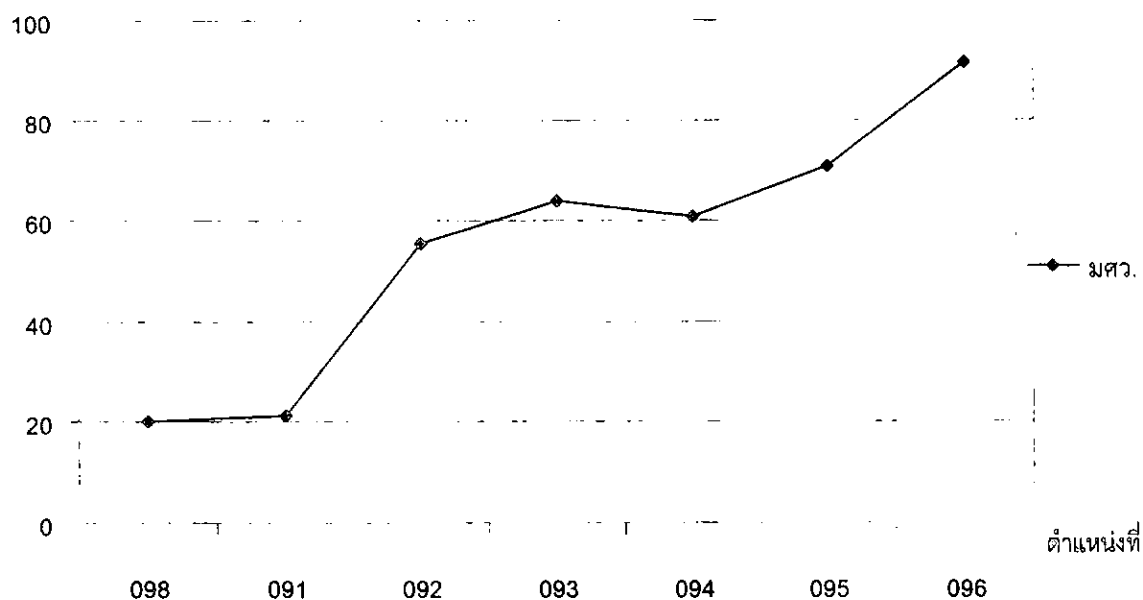
กราฟที่ 17 ปริมาณคลอรีนในน้ำคลองแสนแสบในเดือนธันวาคม 2543
