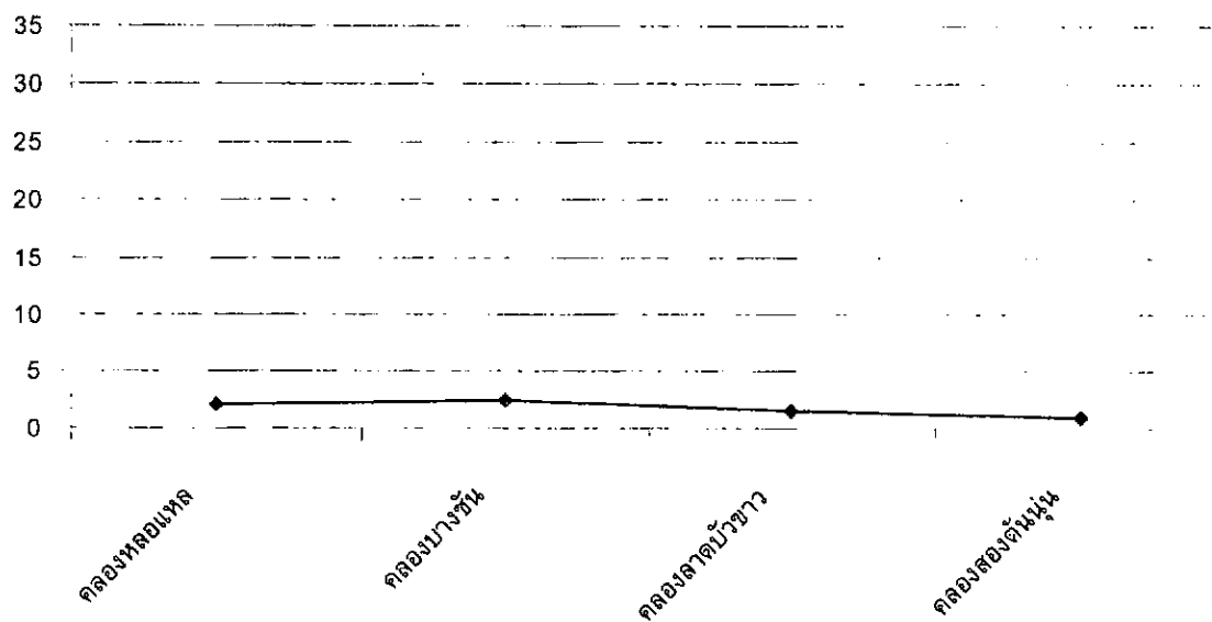
กราฟที่ 51 ปริมาณที่ เค เอ็นในน้ำคลองย่อย 4 คลอง ในเดือนพฤษภาคม 2544
