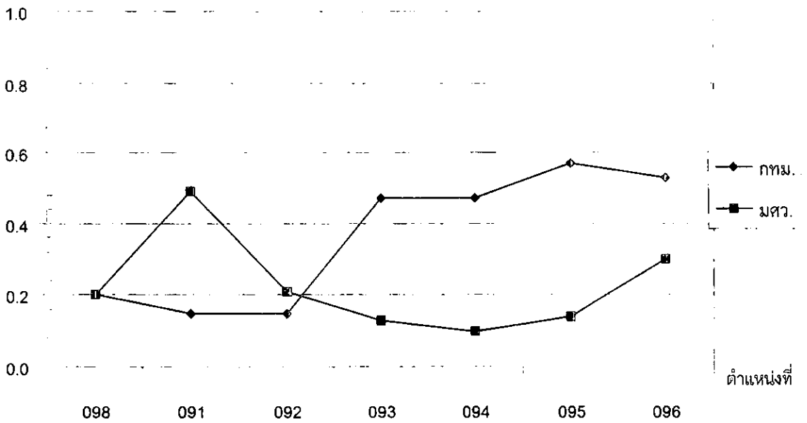
กราฟที่ 22 ปริมาณไนเตรตในหน่วยไนโตรเจนในน้ำคลองแสนแสบในระหว่าง เดือนมกราคม - มีนาคม 2544
