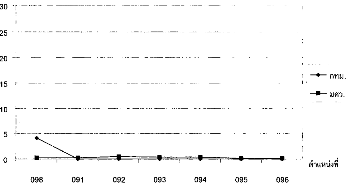
กราฟที่ 28 ปริมาณแอมโมเนียในหน่วยไนโตรเจนในน้ำคลองแสนแสบในระหว่าง เดือนกรกฎาคม - กันยายน 2544
