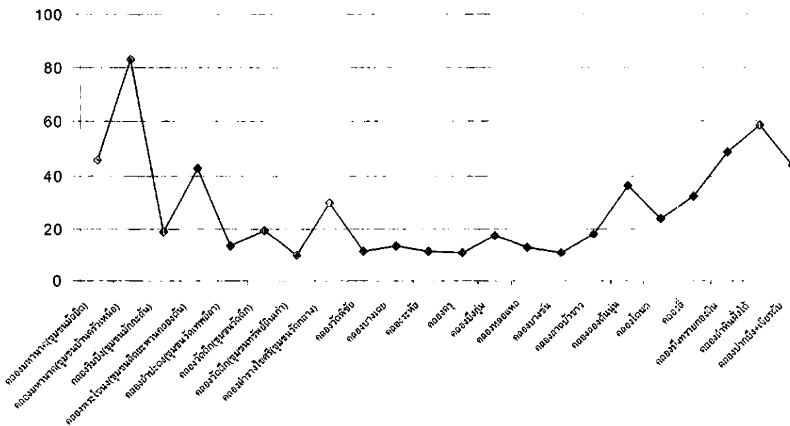
กราฟที่ 62 ปริมาณของแข็งแขวนลอยทั้งหมดในน้ำคลองย่อย 22 คลอง ในเดือนพฤศจิกายน 2544
