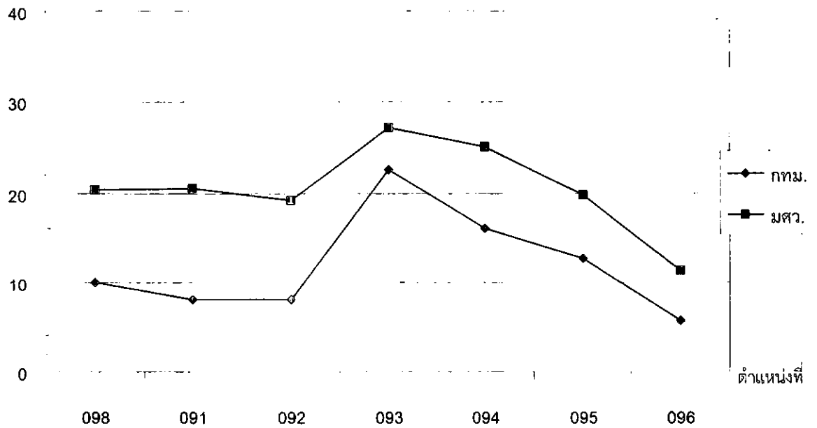
กราฟที่ 6 ปริมาณน้ำใช้ดีในน้ำคลองแสนแสบในระหว่างเดือนมกราคม - มีนาคม 2544
