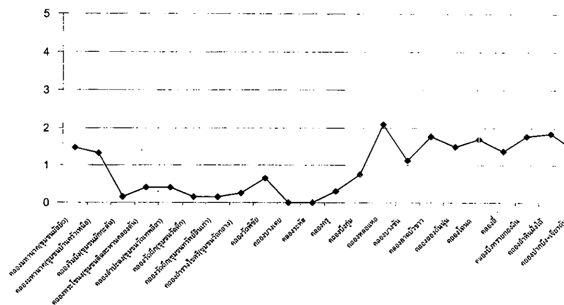
กราฟที่ 56 ปริมาณออกซิเจนละลายในน้ำคลองย่อย 22 คลอง ในเดือนพฤศจิกายน 2544
