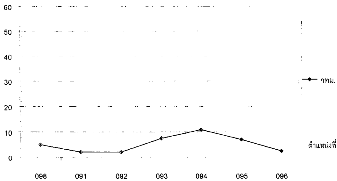
กราฟที่ 29 ปริมาณที่ เค เอ็นในน้ำคลองแสนแสบในเดือนธันวาคม 2543
