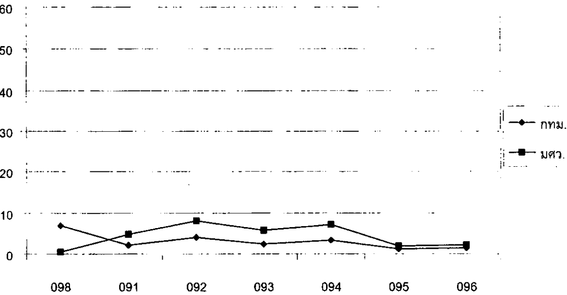
กราฟที่ 32 ปริมาณที่ เค เอ็นในน้ำคลองแสนแสบในระหว่างเดือนกรกฎาคม – กันยายน 2544
