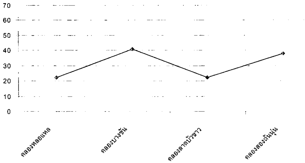
กราฟที่ 41 ปริมาณน้ำดีในน้ำคลองย่อย 4 คลอง ในเดือนพฤษภาคม 2544
