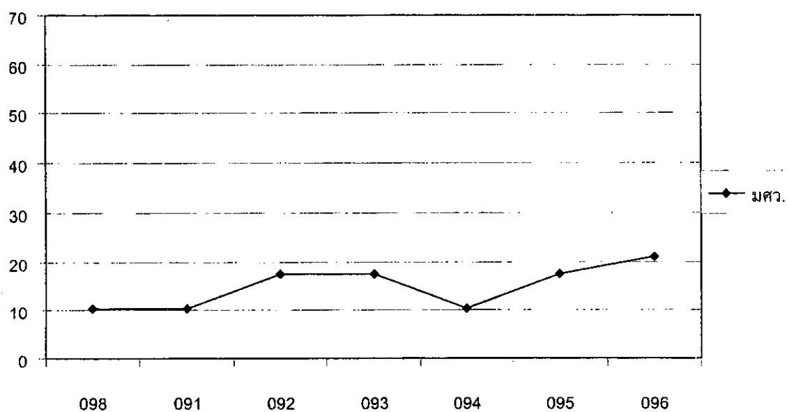
กราฟที่ 12 ปริมาณไนไตรต์ในน้ำคลองแสนแสบในระหว่างเดือนกรกฎาคม - กันยายน 2544
