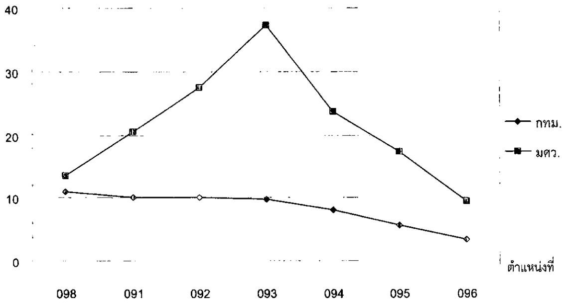
กราฟที่ 5 ปริมาณน้ำใช้ดีในน้ำคลองแสนแสบในเดือนธันวาคม 2543
