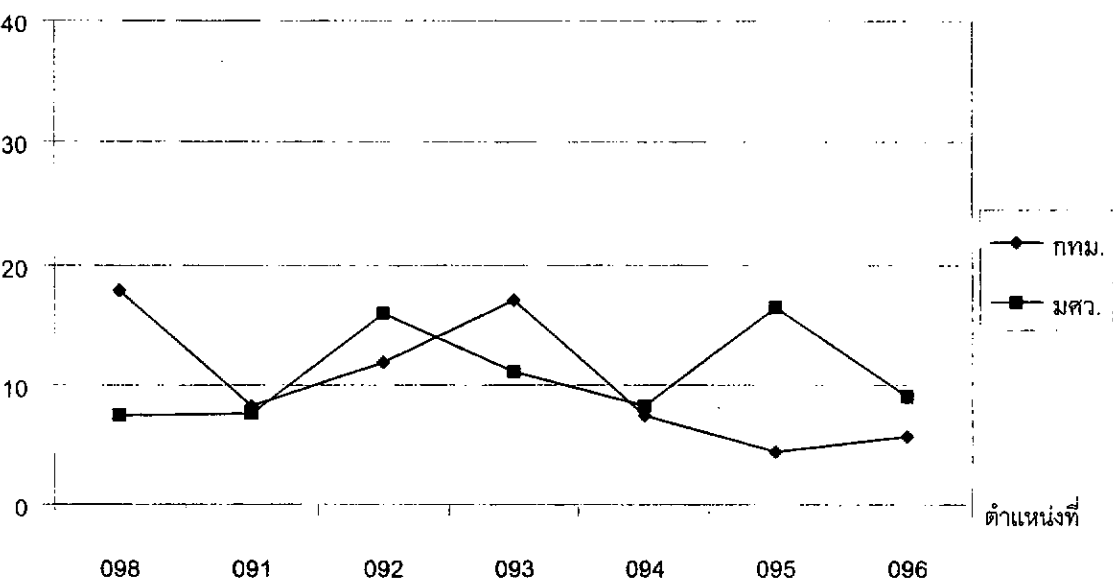
กราฟที่ 8 ปริมาณไนไตรต์ในน้ำคลองแสนแสบในระหว่างเดือนกรกฎาคม – กันยายน 2544
