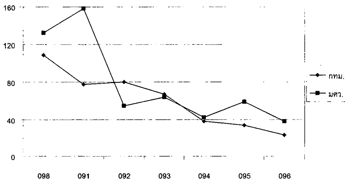
กราฟที่ 16 ปริมาณของแข็งแขวนลอยทั้งหมดในน้ำคลองแสนแสบในระหว่างเดือนกรกฎาคม – กันยายน 2544
