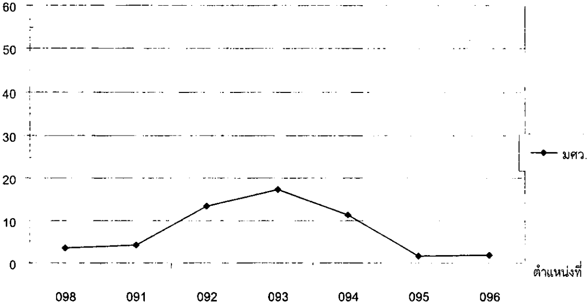
กราฟที่ 31 ปริมาณที่ เค เอ็นในน้ำคลองแสนแสบในระหว่างเดือนเมษายน – มิถุนายน 2544
