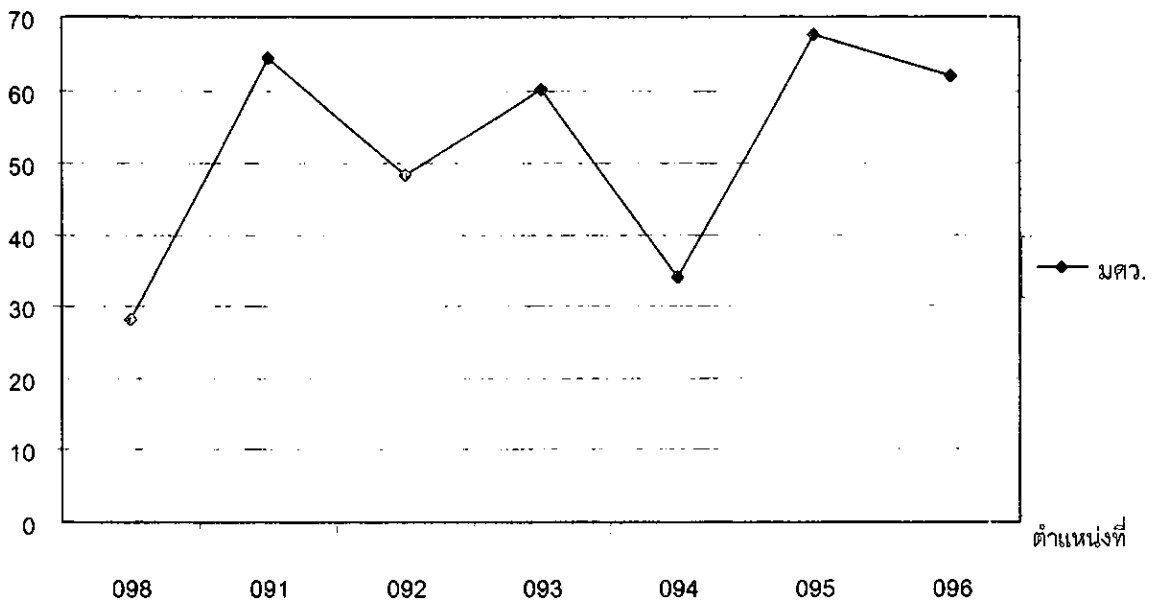
กราฟที่ 10 ปริมาณซีไอดีในน้ำคลองแสนแสบในระหว่างเดือน มกราคม – มีนาคม 2544
