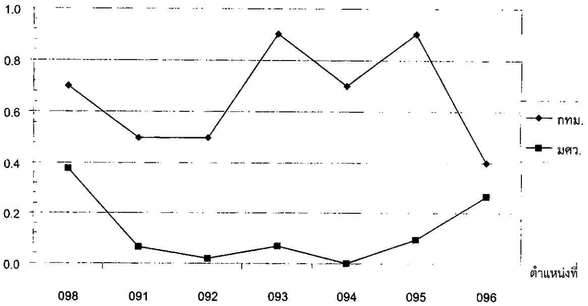
กราฟที่ 23 ปริมาณไนเตรตในหน่วยไนโตรเจนในน้ำคลองแสนแสบในระหว่าง เดือนเมษายน - มิถุนายน 2544
