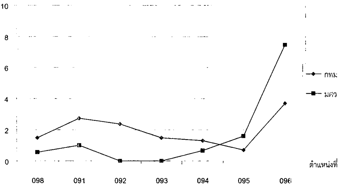
กราฟที่ 1 ปริมาณออกซิเจนละลายน้ำในคลองแสนแสบในเดือนธันวาคม 2543
