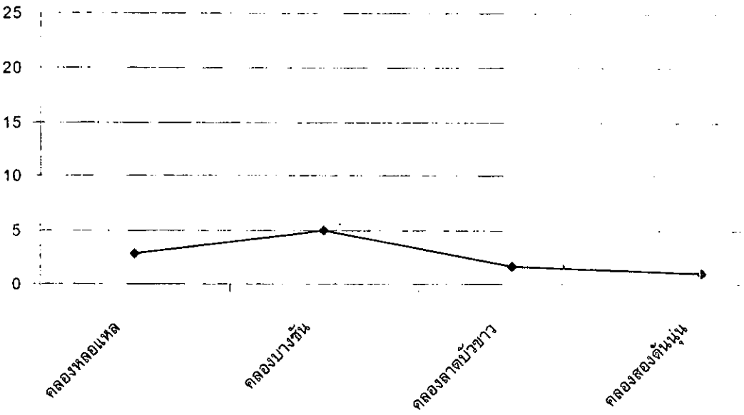
กราฟที่ 39 ปริมาณบีโอดีในน้ำคลองย่อย 4 คลอง ในเดือนพฤษภาคม 2544
