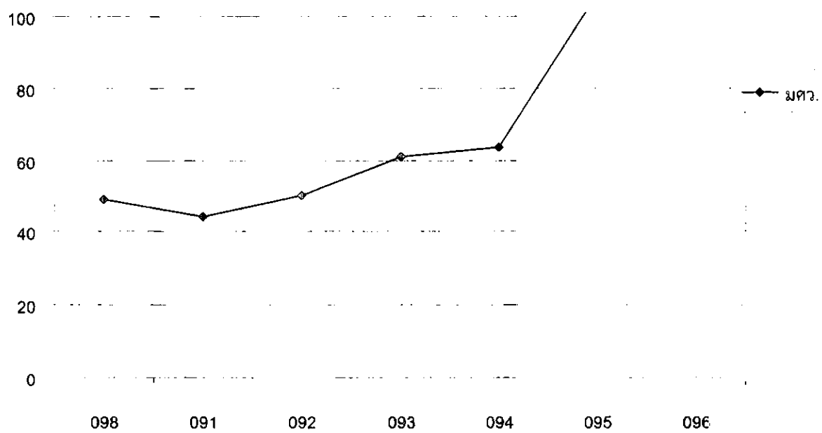
กราฟที่ 18 ปริมาณคลอรีนในน้ำคลองแสนแสบในระหว่างเดือนมกราคม – มีนาคม 2544
