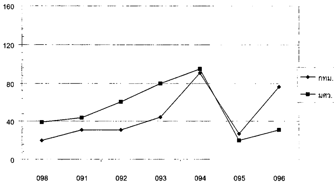
กราฟที่ 15 ปริมาณของแข็งแขวนลอยทั้งหมดในน้ำคลองแสนแสบในระหว่างเดือนเมษายน – มิถุนายน 2544
