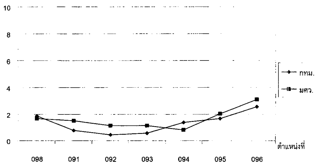
กราฟที่ 4 ปริมาณออกซิเจนละลายน้ำในคลองแสนแสบในระหว่างเดือนกรกฎาคม – กันยายน 2544
