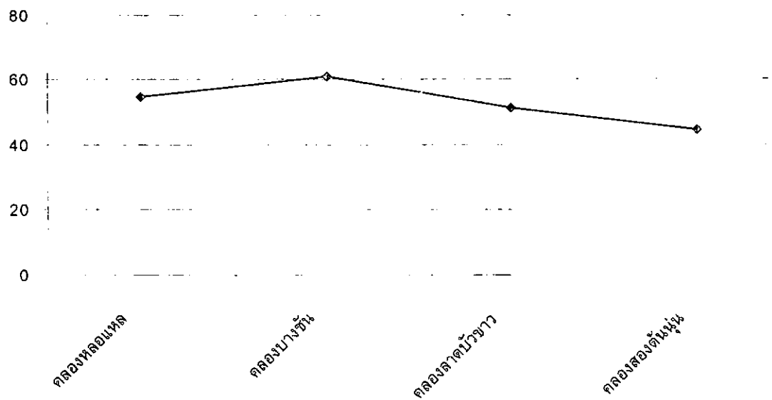
กราฟที่ 45 ปริมาณคลอรีนในน้ำคลองย่อย 4 คลอง ในเดือนพฤษภาคม 2544
