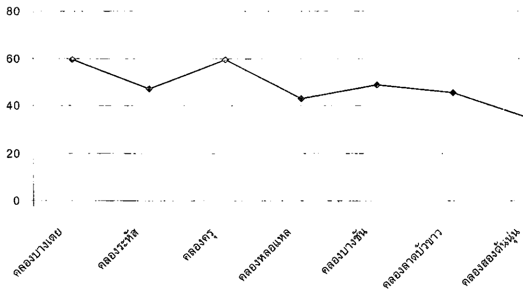
กราฟที่ 46 ปริมาณคลอรีนในน้ำคลองย่อย 7 คลอง ในเดือนกรกฎาคม 2544
