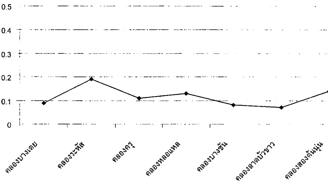
กราฟที่ 48 ปริมาณไนเตรตในหน่วยไนโตรเจนในน้ำคลองย่อย 7 คลอง ในเดือนกรกฎาคม 2544
