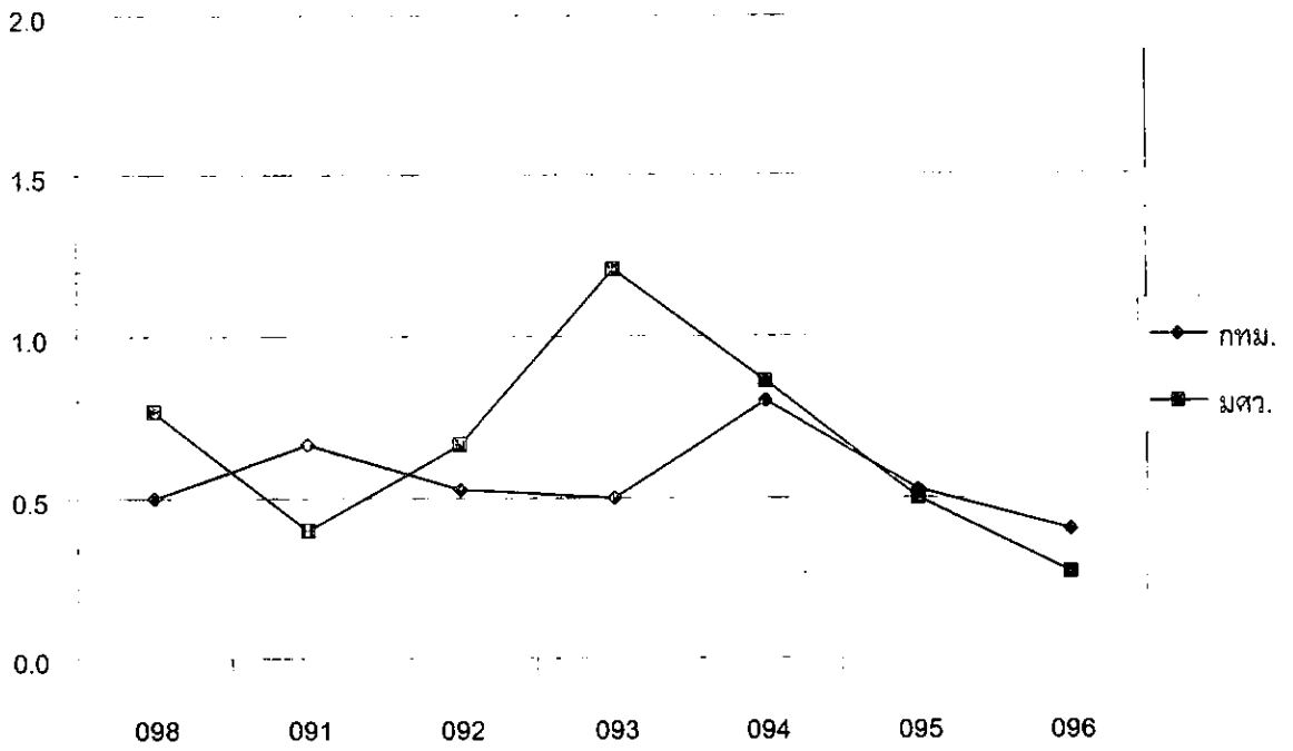
กราฟที่ 33 ปริมาณฟอสฟอรัสทั้งหมดในน้ำคลองแสนแสบในเดือนธันวาคม 2543
