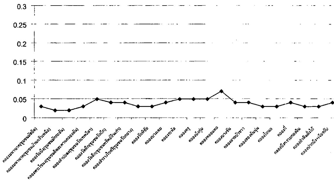
กราฟที่ 67 ปริมาณแอมโมเนียในหน่วยไนโตรเจนในน้ำคลองย่อย 22 คลอง ในเดือนตุลาคม 2544
