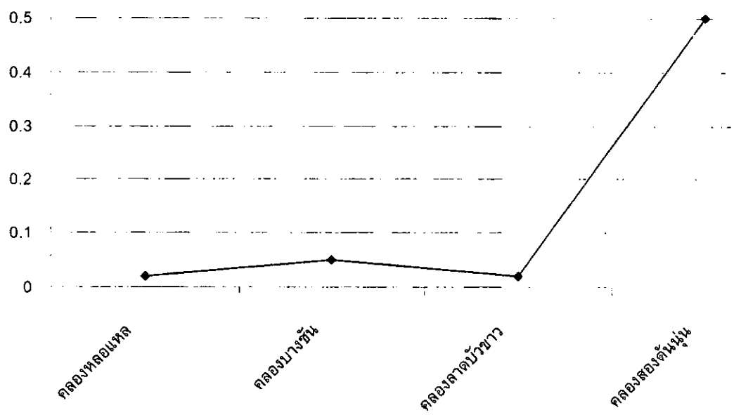
กราฟที่ 47 ปริมาณไนเตรตในหน่วยไนโตรเจนในน้ำคลองย่อย 4 คลอง ในเดือนพฤษภาคม 2544
