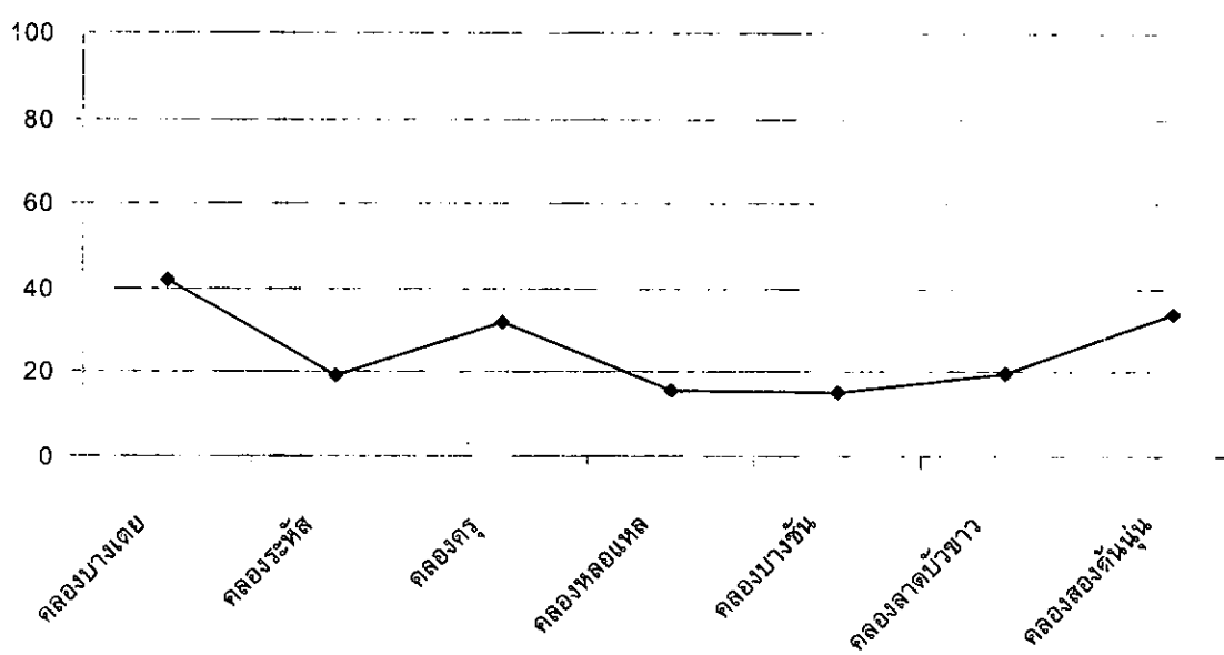
กราฟที่ 44 ปริมาณของแข็งแขวนลอยทั้งหมดในน้ำคลองย่อย 7 คลอง ในเดือนกรกฎาคม 2544
