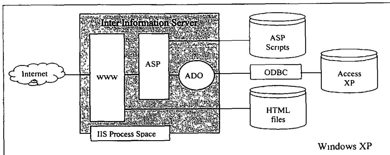
ภาพประกอบ 2 การทำงานของเอเอสพี ร่วมกับฐานข้อมูลโดยผ่าน เอดีโอ
