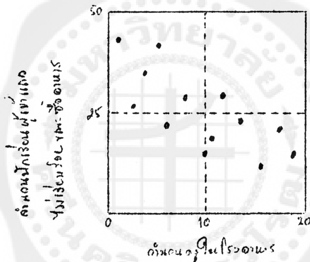
แผนภูมิควบคุม
