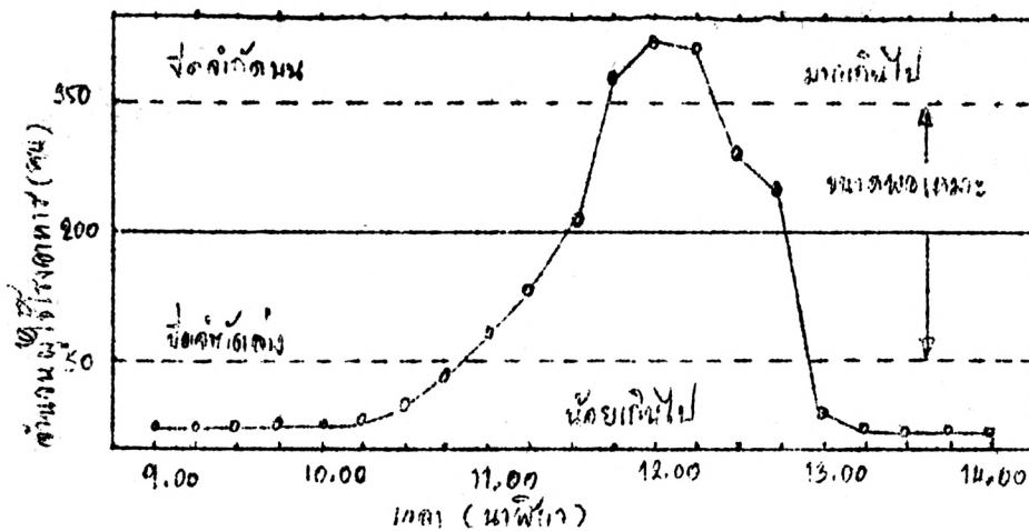
แผนภูมิควบคุม
