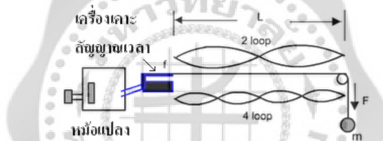
รูป 13 ชุดทดลองคลื่นนิ่งบนเส้นเชือกที่นิยมใช้ในระดับโรงเรียนทั่วไป
