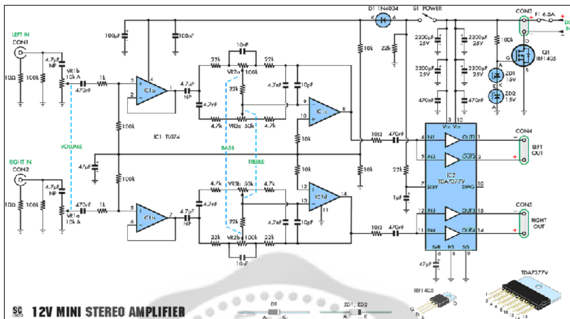
รูป 19 วงจรอิเล็กทรอนิกส์ของเครื่องขยายกำลัง
