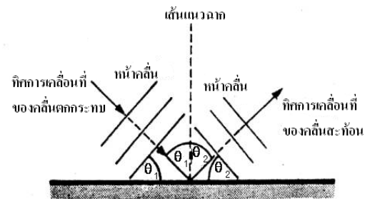
รูป 6 ทิศทางการเคลื่อนที่ของคลื่น
