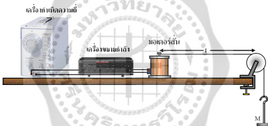
รูป 14 ชุดทดลองคลื่นนิ่งบนเส้นเชือกรูปแบบที่ 2
