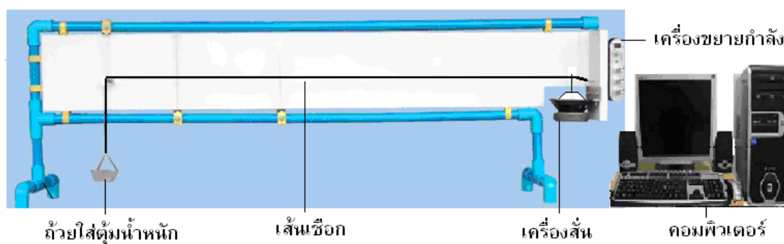
รูป 22 ชุดทดลองคลื่นนิ่งบนเส้นเชือกที่พัฒนาขึ้น
