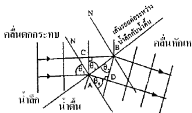
รูป 7 การหักเหของคลื่น
