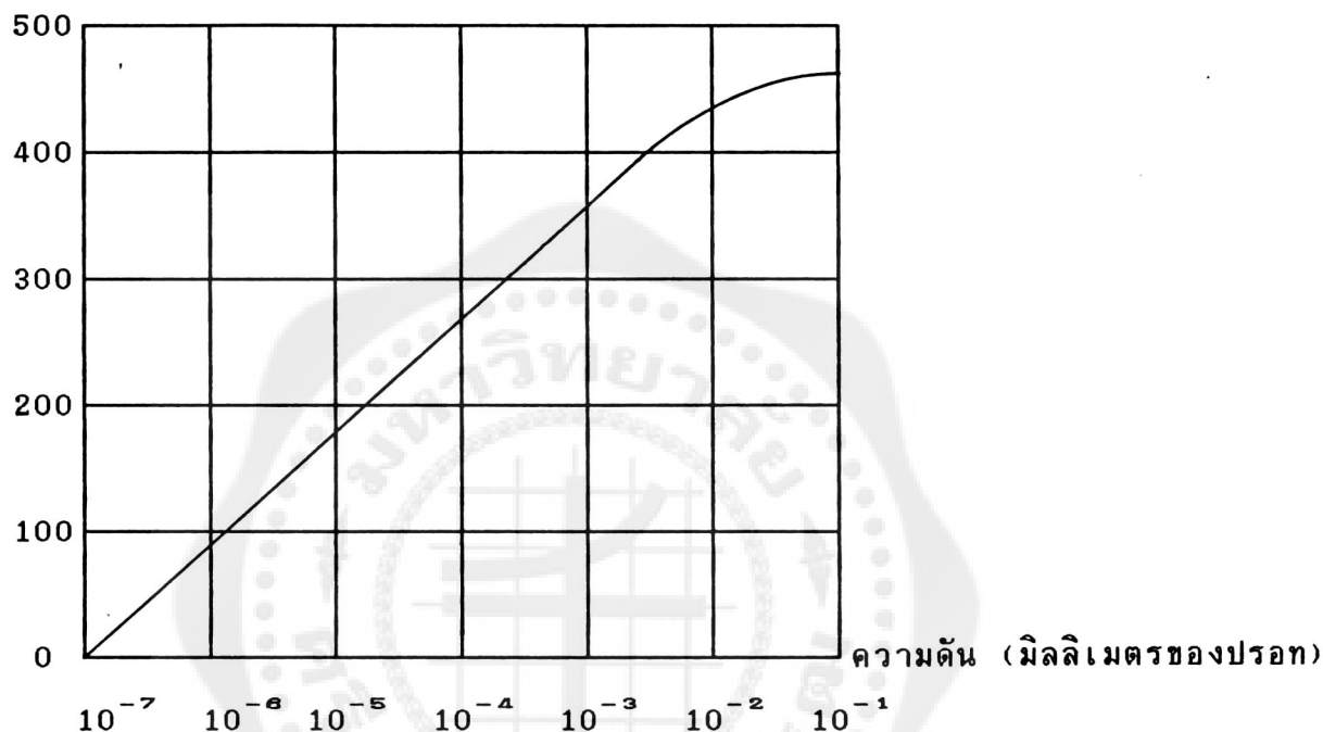
รูปที่ 1.10 กราฟแสดงความสัมพันธ์ระหว่างกระแสและความดันของเครื่องวัดแบบเพนนิ่ง
