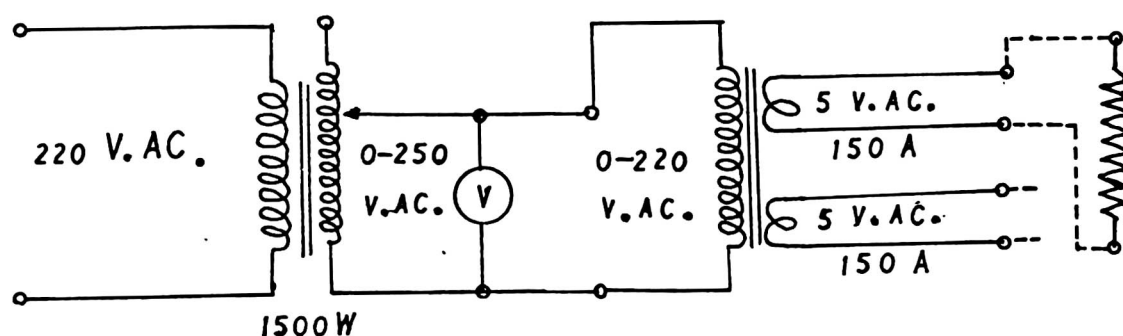
รูปที่ 2.41 การต่อวงจรไฟฟ้าของหม้อแปลงไฟฟ้าชนิดกระแสสูงความต่างศักย์ต่ำสำหรับลวดความร้อนระเหยสาร
