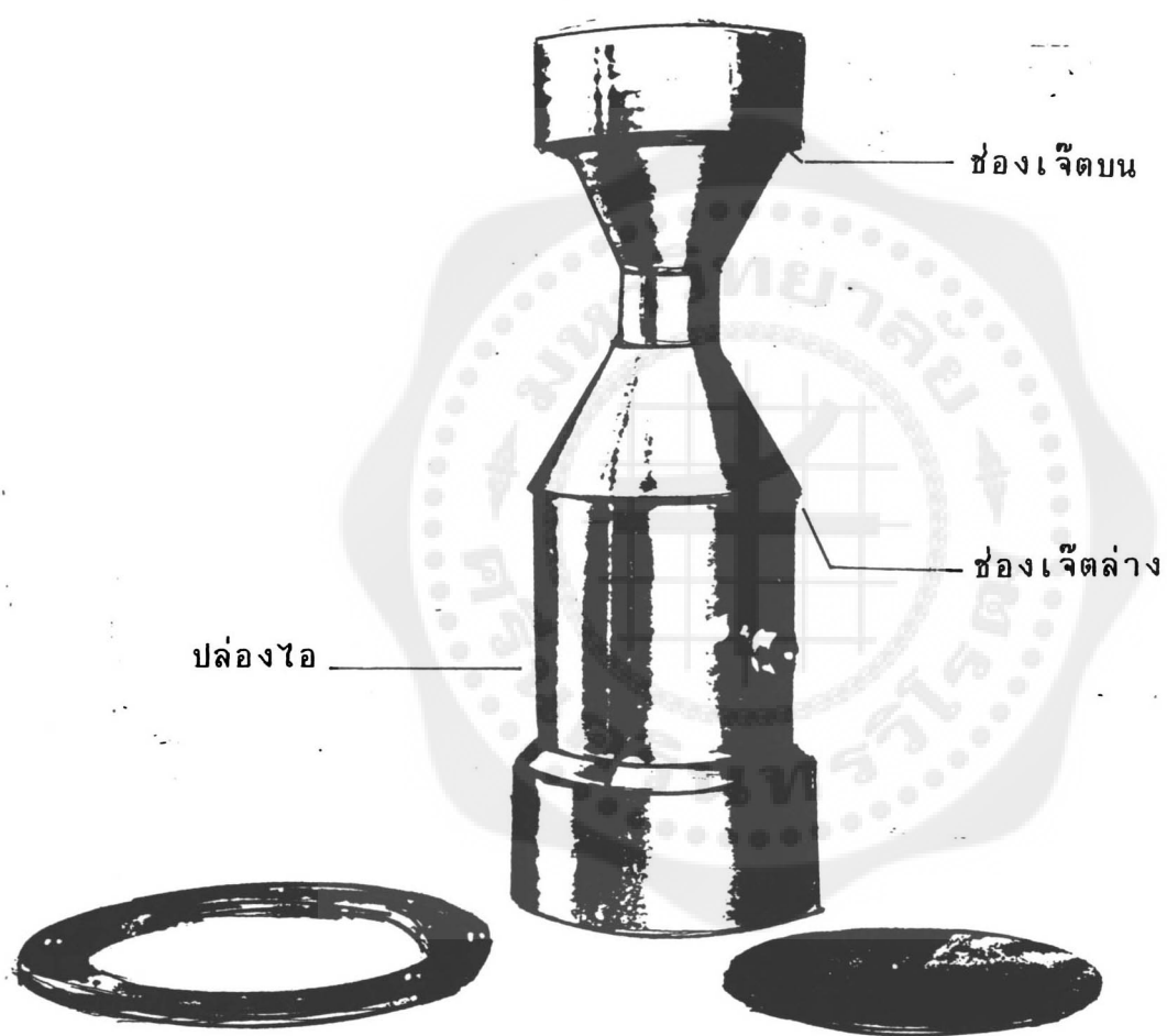
รูปที่ 2.10 แสดงการประกอบชิ้นส่วนในรูปที่ 2.9 ให้เป็นปล่องไอและท่อเจ็ต ในรูปยังแสดงฐานยึดจากกำบังและฝาจากกำบัง
