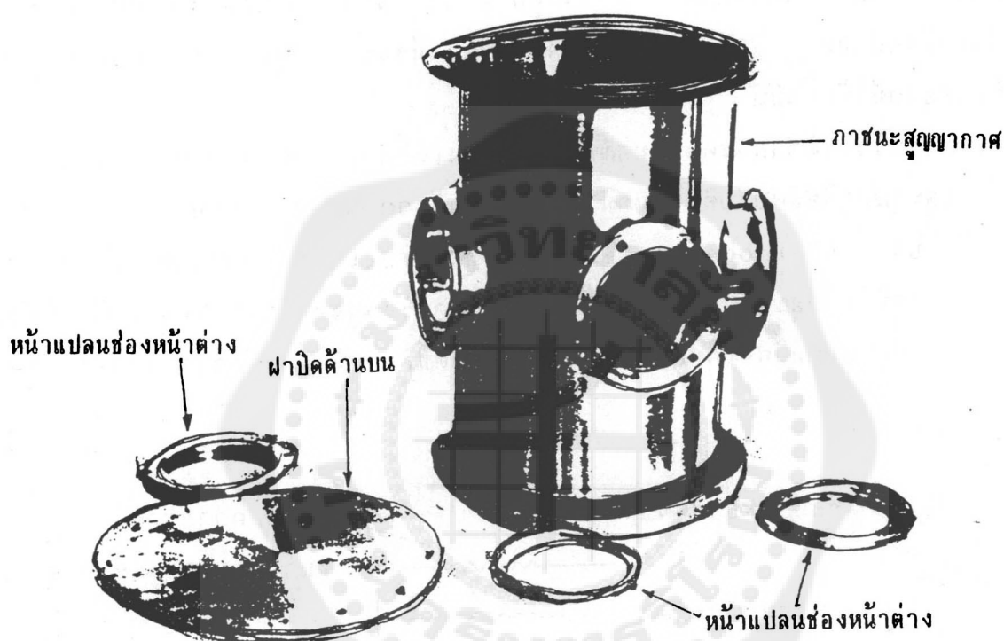
รูปที่ 2.13 ภาชนะสุญญากาศที่สร้างขึ้น แสดงให้เห็นแผ่นปิดด้านบน และวงแหวนยึดกระจกที่ช่องมอง
