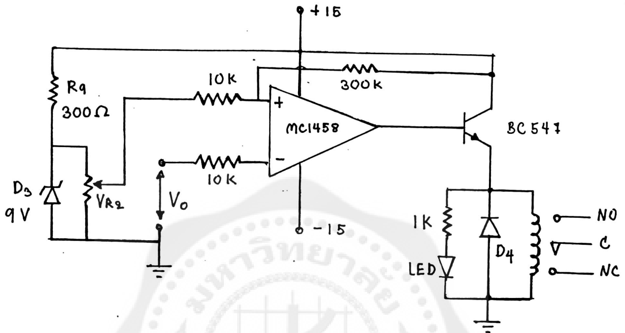
รูปที่ 2.28 วงจรควบคุมอุปกรณ์ภายนอก
