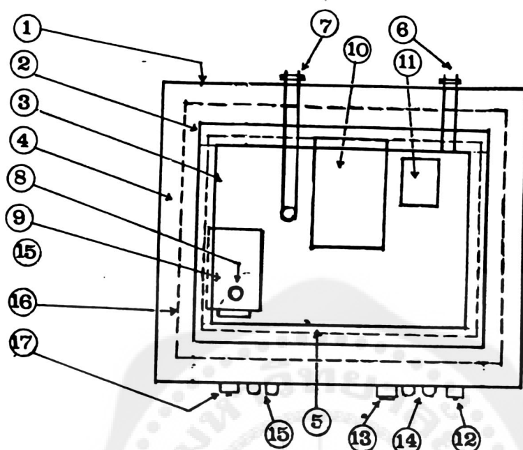
ค. ภาพแสดงภาคตัดด้านบนของเครื่องทำน้ำเย็น
