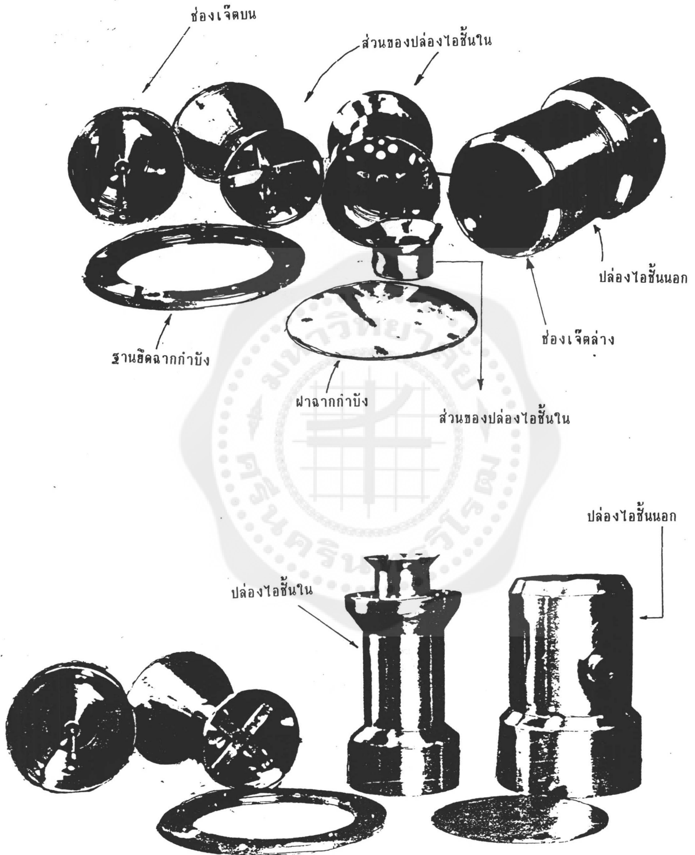
รูปที่ 2.9 ชิ้นส่วนภายในของเครื่องสุญญากาศแบบแพร่ไอที่สร้างขึ้น
