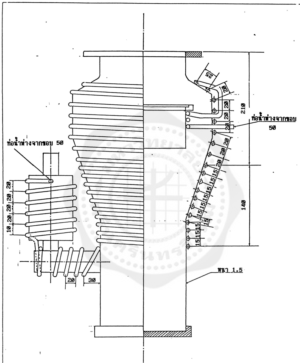
รูปที่ 2.4 แบบการพันท่อทองแดงเพื่อใช้เป็นท่อระบายความร้อน
