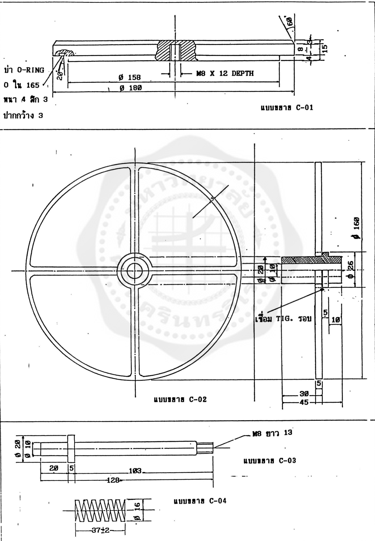
รูปที่ 2.16 ส่วนขยายแบบด้านล่างของแผ่นฐาน
