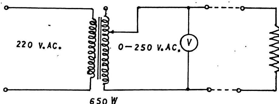
รูปที่ 2.43 แสดงการต่อวงจรไฟฟ้าระหว่างหม้อแปลงไฟฟ้าปรับค่าได้กับขดลวดความร้อนอบชิ้นงาน
