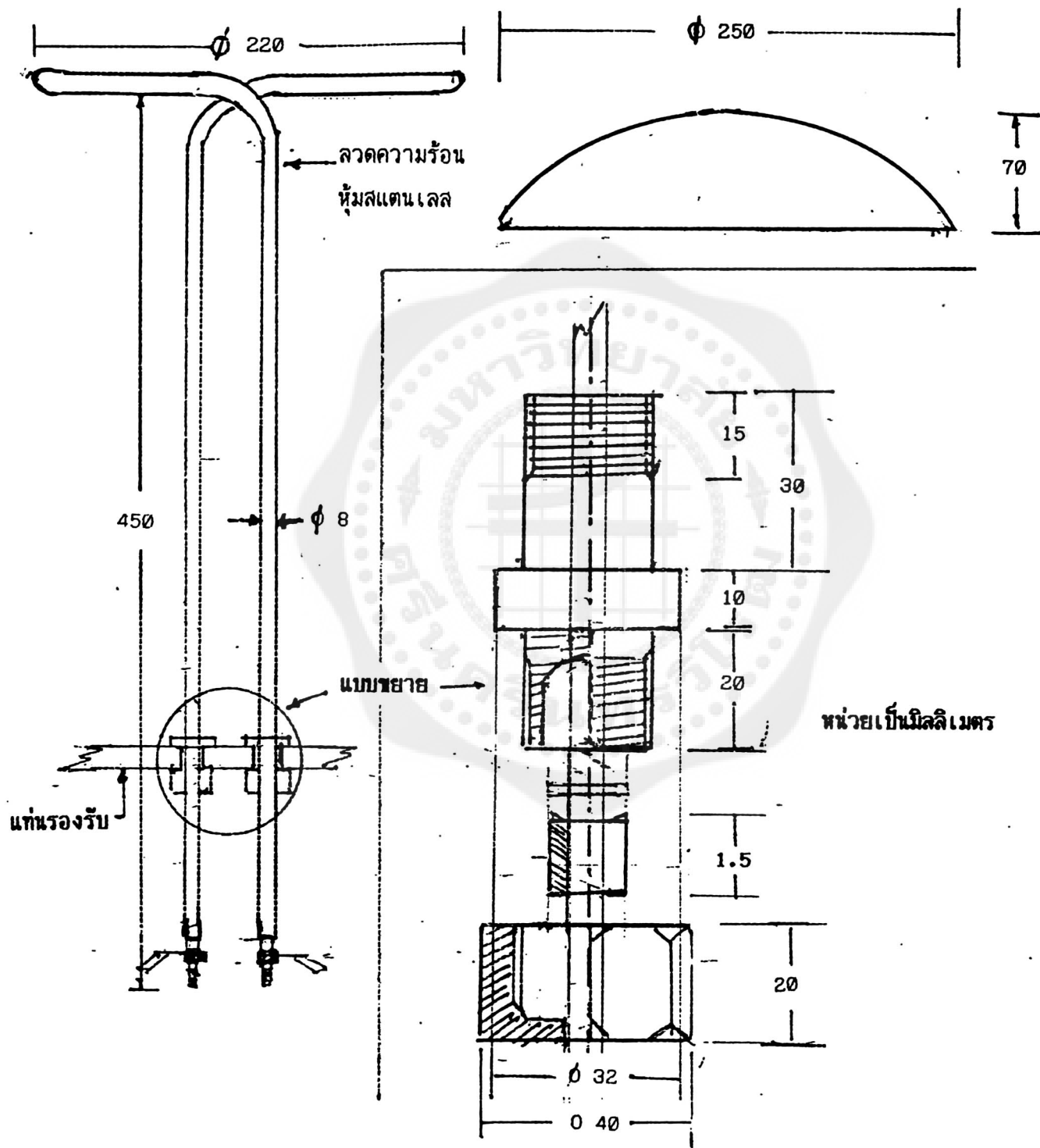
รูปที่ 2.35 แบบระบบอบชิ้นงาน
