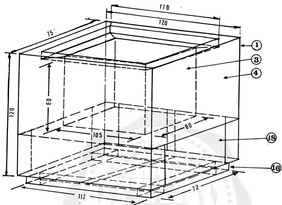
ก. ภาพแสดงโครงสร้างของเครื่องทำน้ำเย็น
