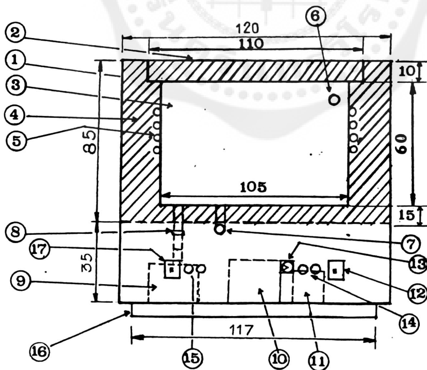
ง. ภาพแสดงภาคตัดด้านหน้าของเครื่องทำน้ำเย็น
