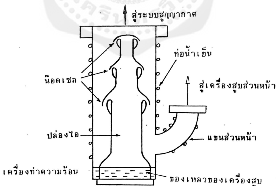
รูปที่ 1.5 เครื่องสูบน้ำอากาศแบบแพร่ไอ
