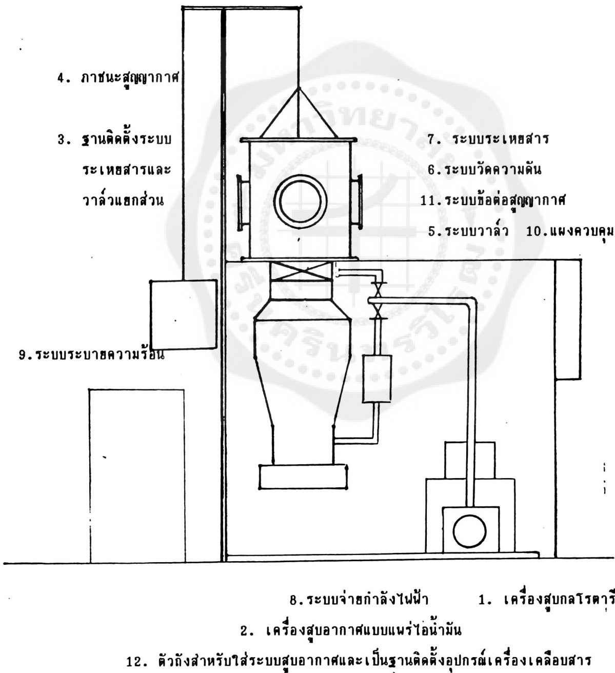
รูปที่ 2.1 แผนภาพของเครื่องเคลือบสารระบบสุญญากาศที่สร้างขึ้น
