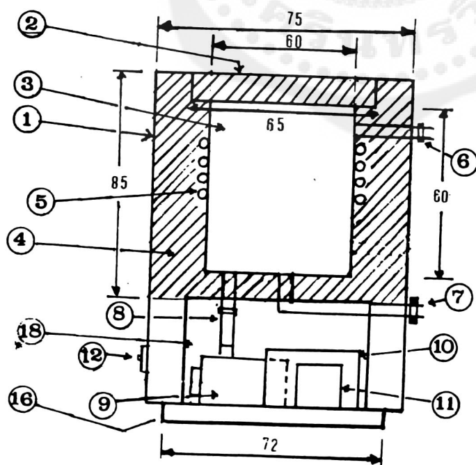
ข. ภาพแสดงภาคตัดด้านข้างของเครื่องทำน้ำเย็น
