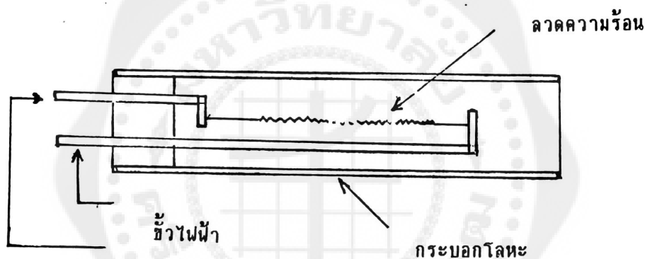
รูปที่ 2.24 โครงสร้างของหัววัดนิรานี
