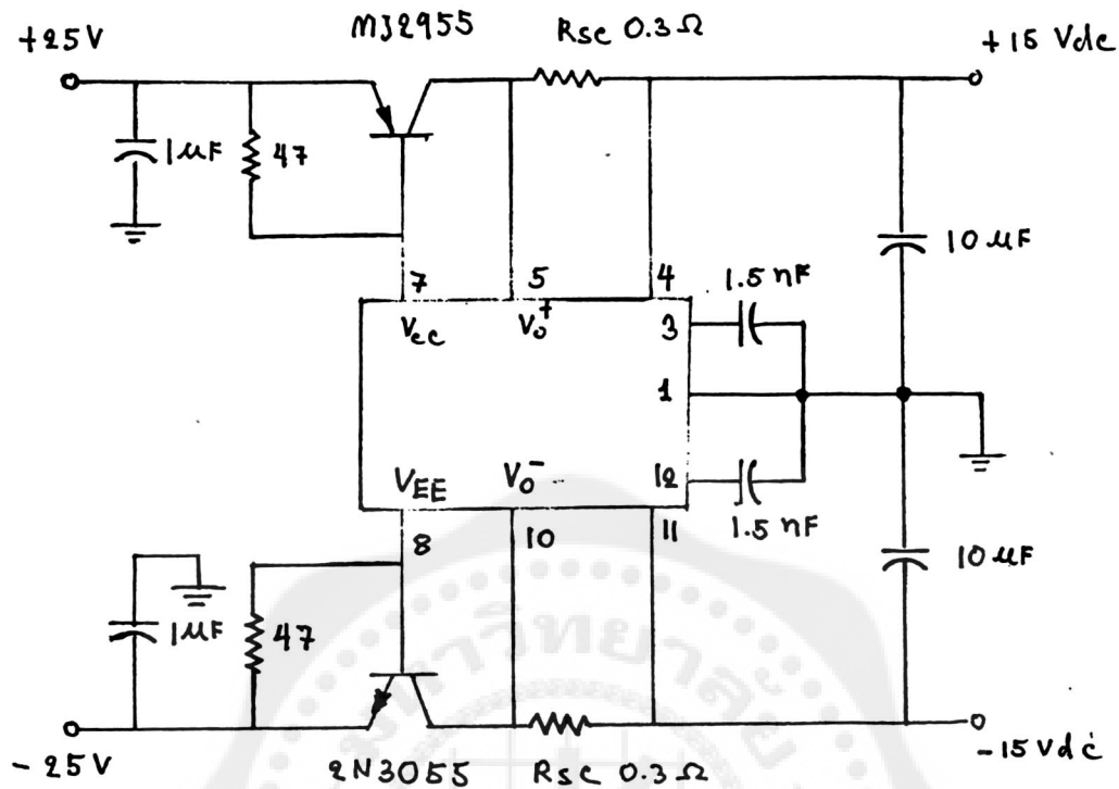
รูปที่ 2.25 รายละเอียดวงจรแหล่งจ่ายไฟกระแสตรง
