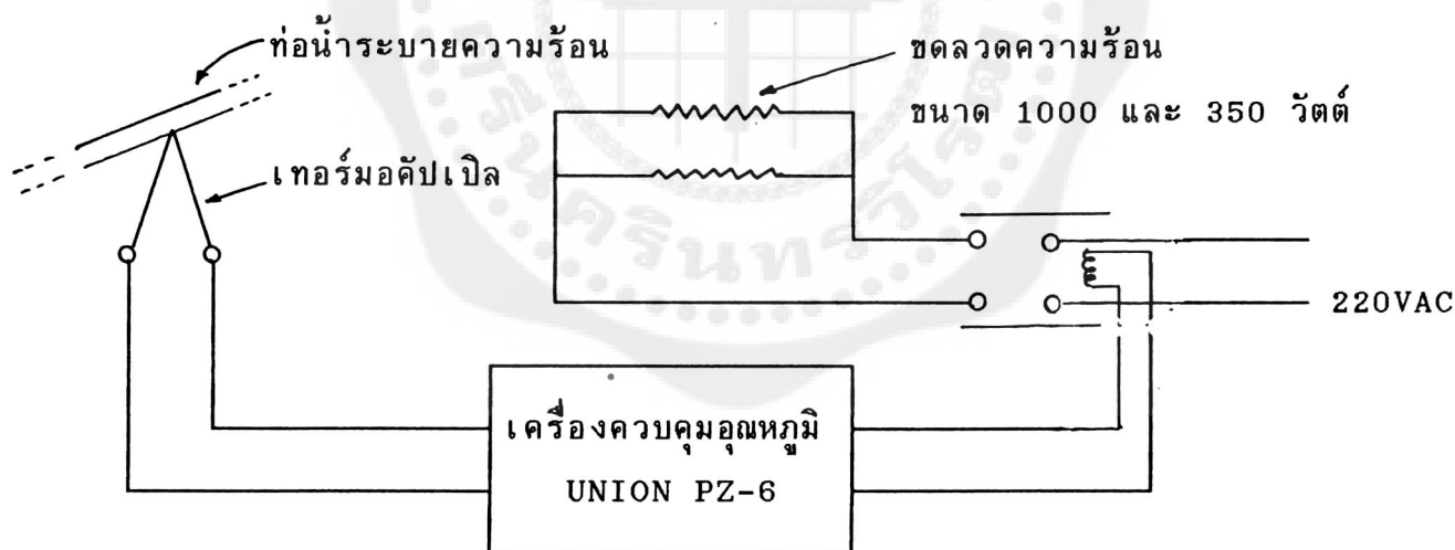
รูปที่ 2.12 วงจรระบบควบคุมอุณหภูมิของน้ำในท่อระบายความร้อน และวงจรไฟฟ้าของขดลวดความร้อนหม้อต้มน้ำมัน
