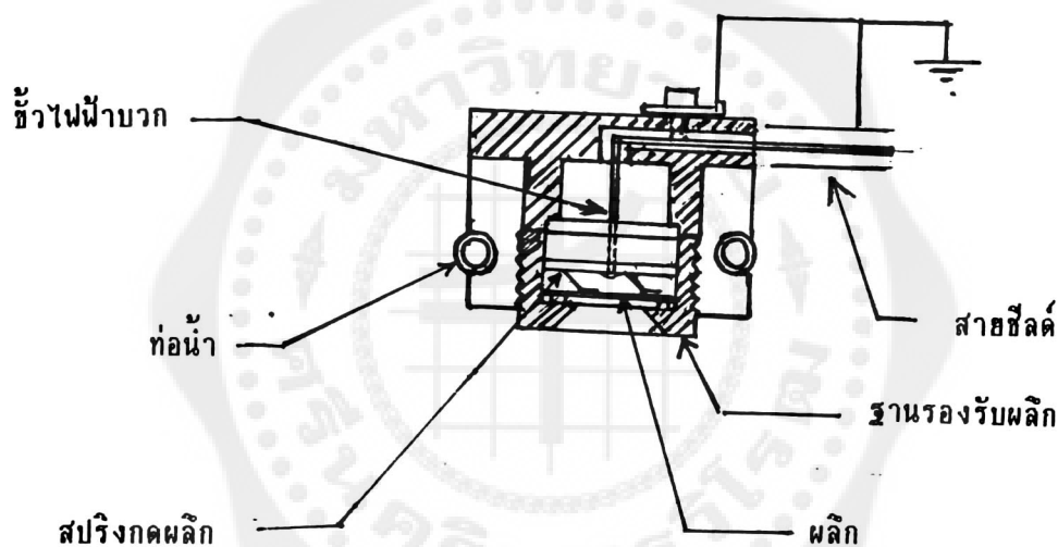
รูป 2.36 ส่วนบนของอุปกรณ์จับผลึก
