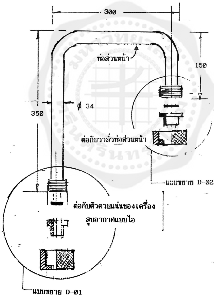
รูปที่ 2.19 แบบท่อส่วนหน้า
