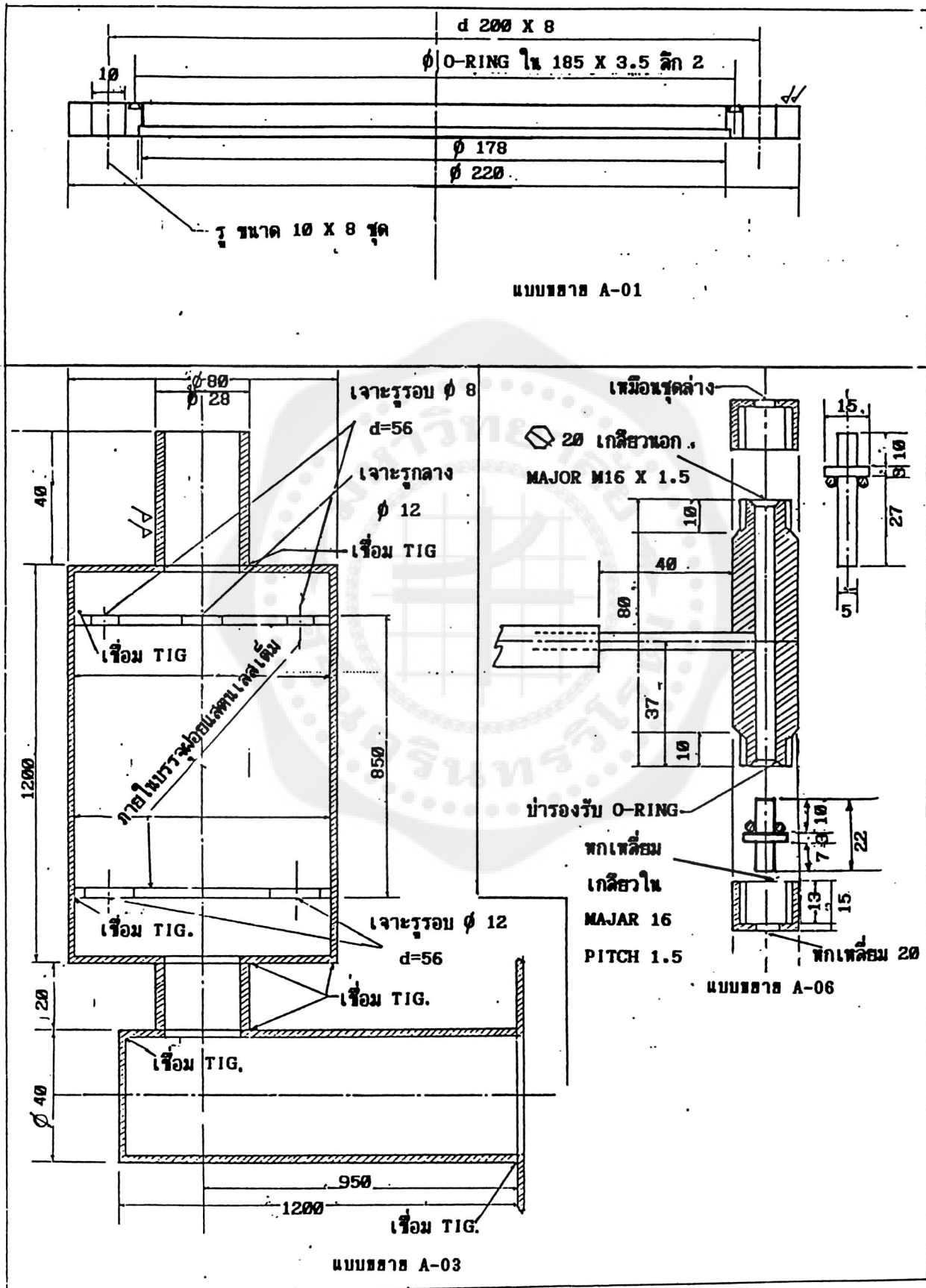
รูปที่ 2.5 ส่วนขยายที่ 1 ของส่วนประกอบภายนอกของเครื่องสูบน้ำแบบแพร่ไอ
