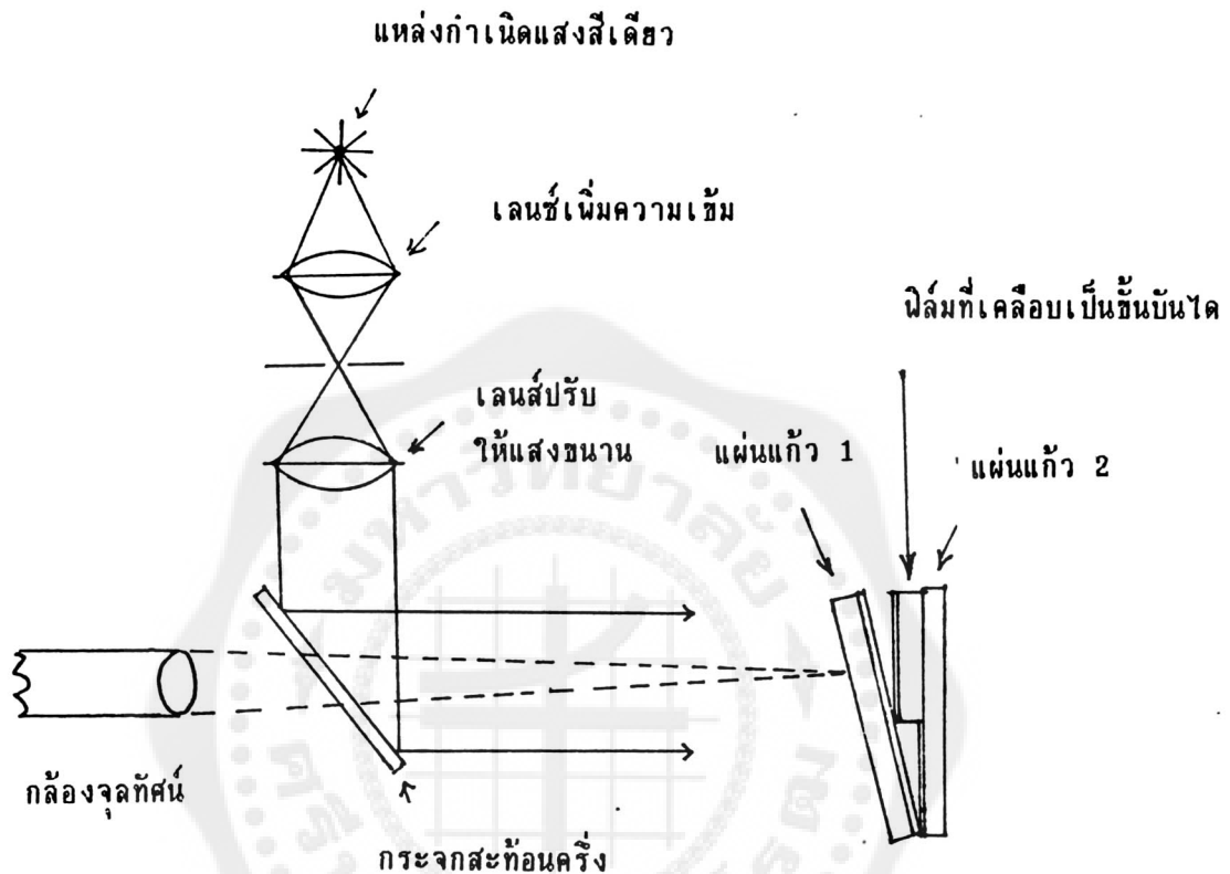
รูปที่ ผ3.1 การจัดวางเครื่องมือการวัดความหนาของฟิล์มด้วยวิธีแทรกสอดของแสง
