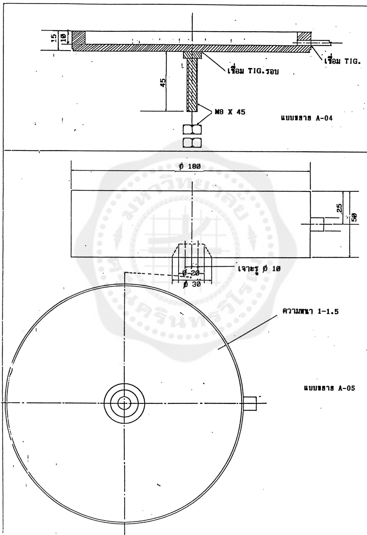
รูปที่ 2.6 ส่วนขยายที่ 2 ของส่วนประกอบภายนอกของเครื่องสุญญากาศแบบแพร่ไอ
