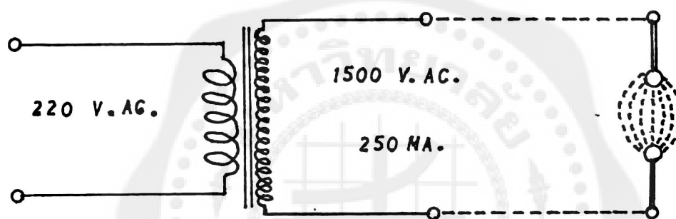
รูปที่ 2.42 การต่อวงจรไฟฟ้าของหม้อแปลงไฟฟ้าความต่างศักย์สูง เข้ากับขั้วไฟฟ้าความต่างศักย์สูงสองขั้ว
