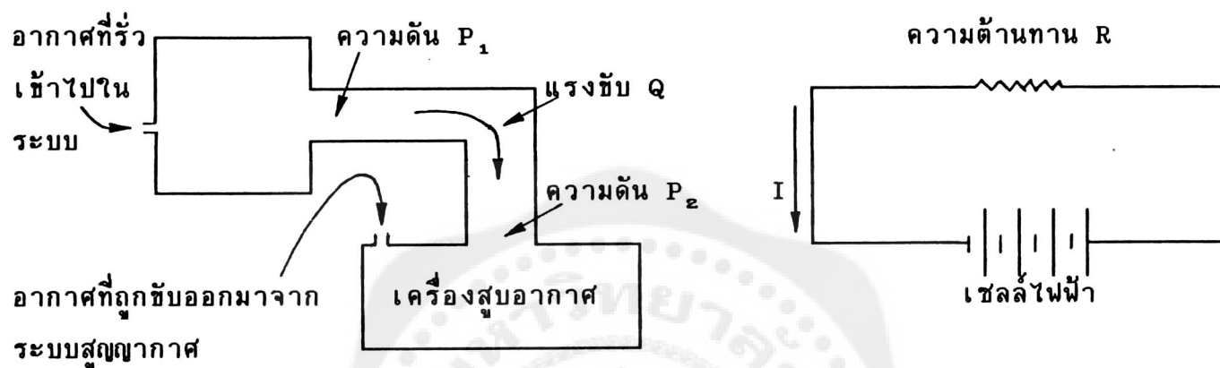
รูปที่ 1.4 การเปรียบเทียบระหว่างระบบสุญญากาศกับวงจรไฟฟ้าอย่างง่าย
