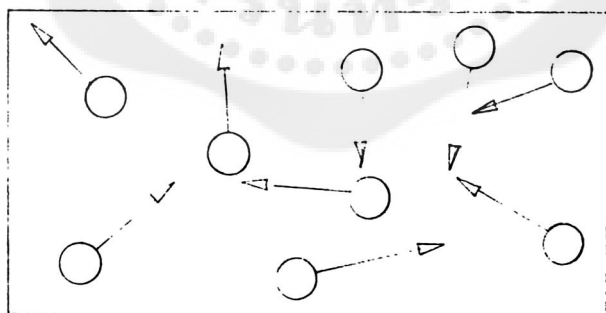
รูปที่ 1.1 การเคลื่อนที่ของโมเลกุลก๊าซในภาชนะปิด
