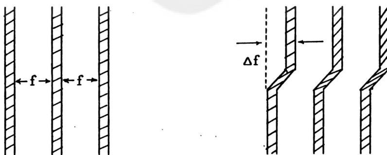
รูปที่ 1.15 ก) รีฟเลกซ์-สว่างในช่วง AB ข) รีฟเลกซ์-สว่างตรงบริเวณ B
