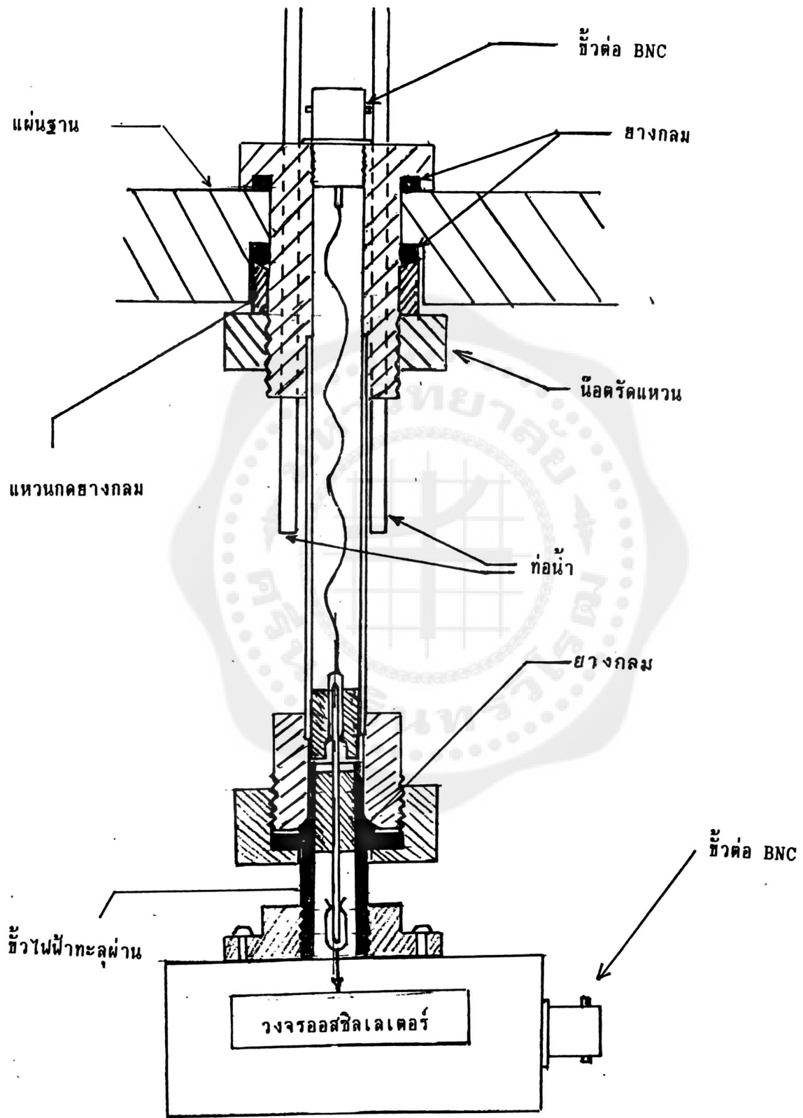
รูปที่ 2.37 ส่วนฐานของอุปกรณ์จับผลึก
