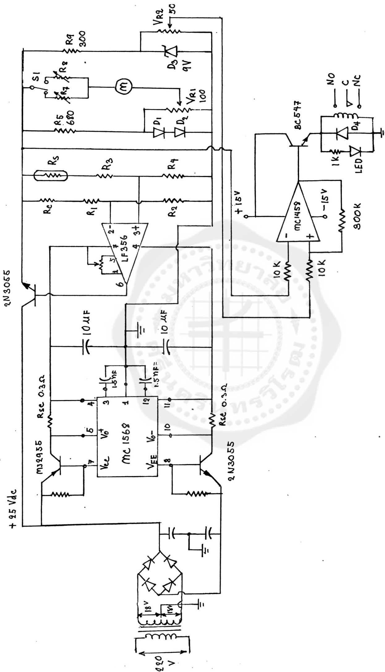
รูปที่ 2.29 วงจรควบคุมความเร็วของมอเตอร์
