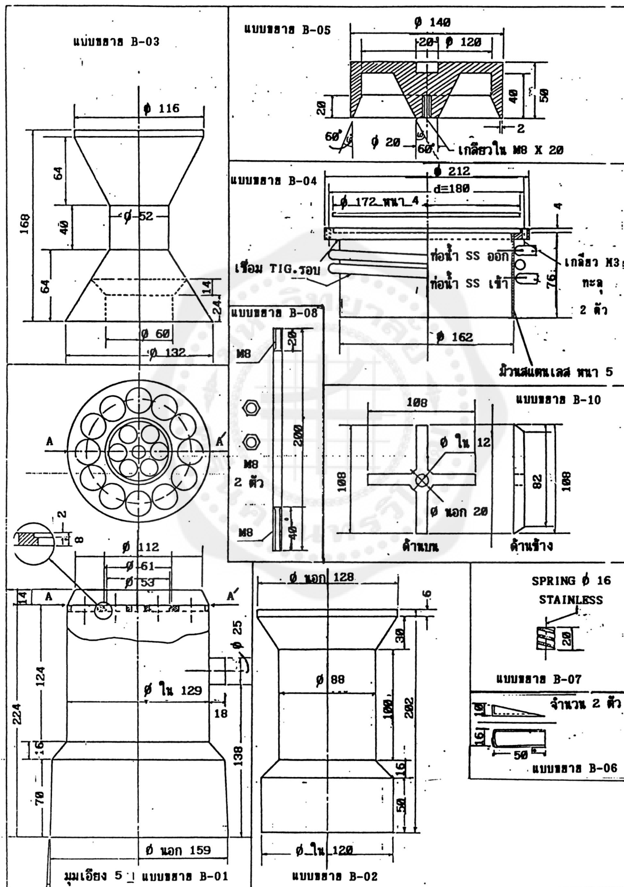
รูปที่ 2.7 ส่วนขยายของแบบของส่วนประกอบภายในของเครื่องสูบน้ำแบบแฟร้งไอ
