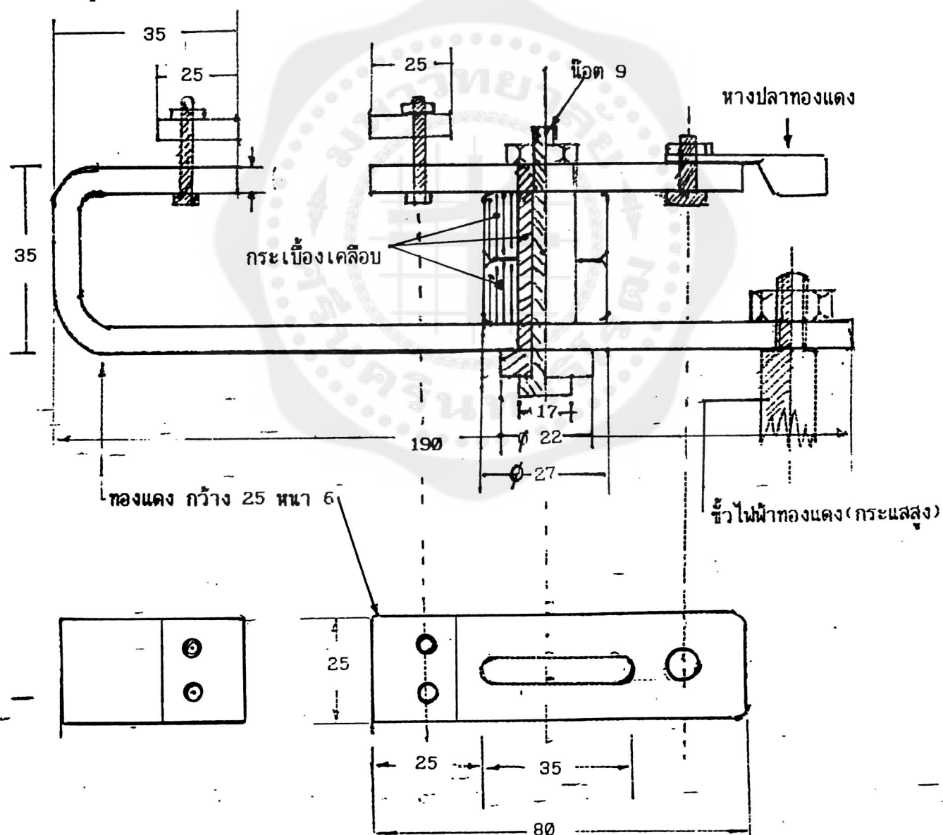
รูปที่ 2.30 แบบขั้วทองแดงจัดยึดโบ๊ต
