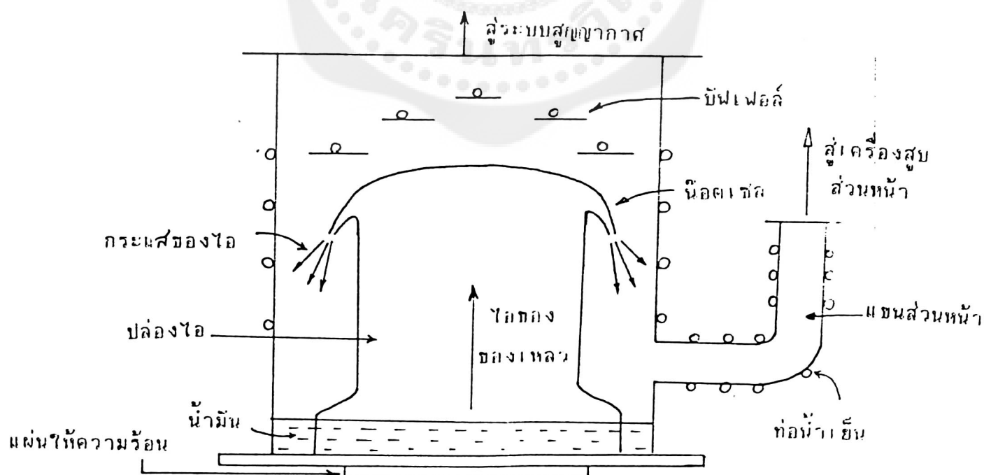
รูปที่ 1.6 โครงสร้างของเครื่องสูบน้ำแบบแพร่ไอ
