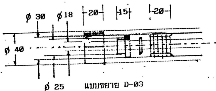
รูปที่ 2.22 ชุดเชื่อมต่อแบบเกลียว
