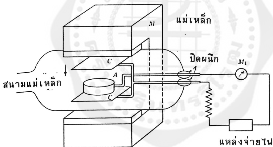
รูปที่ 1.9 การวางตัวของคาโทด อาโนด และ สนามแม่เหล็กในหัววัดของเครื่องวัดแบบเพนนิ่ง
