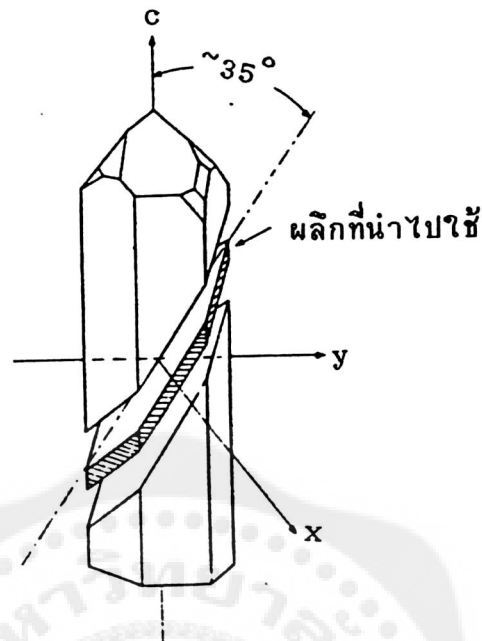
รูปที่ 1.16 การตัดผลึกแบบ AT
