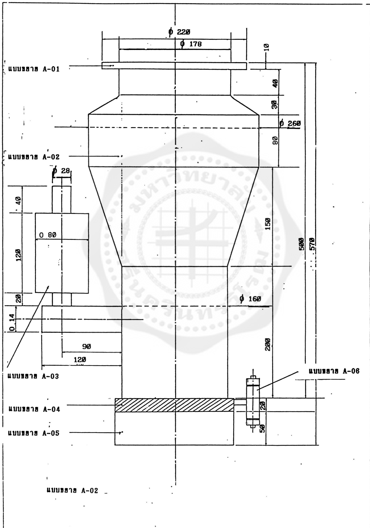
รูปที่ 2.2 แบบส่วนประกอบภายนอกของเครื่องสูบลำอากาศแบบแพร่ไอ
