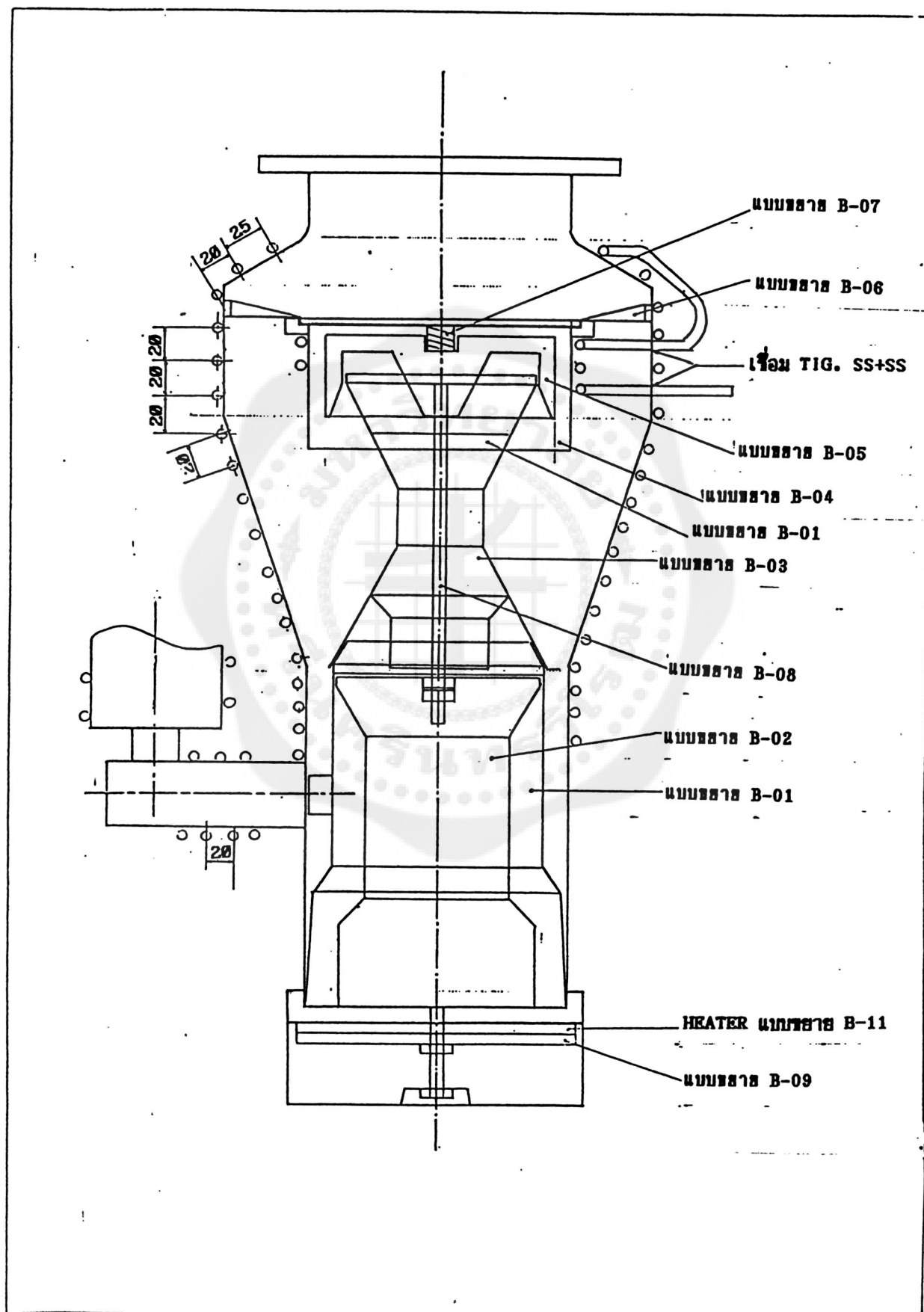
รูปที่ 2.3 แบบส่วนประกอบภายในของเครื่องสูบอากาศแบบแพร่ไอ
