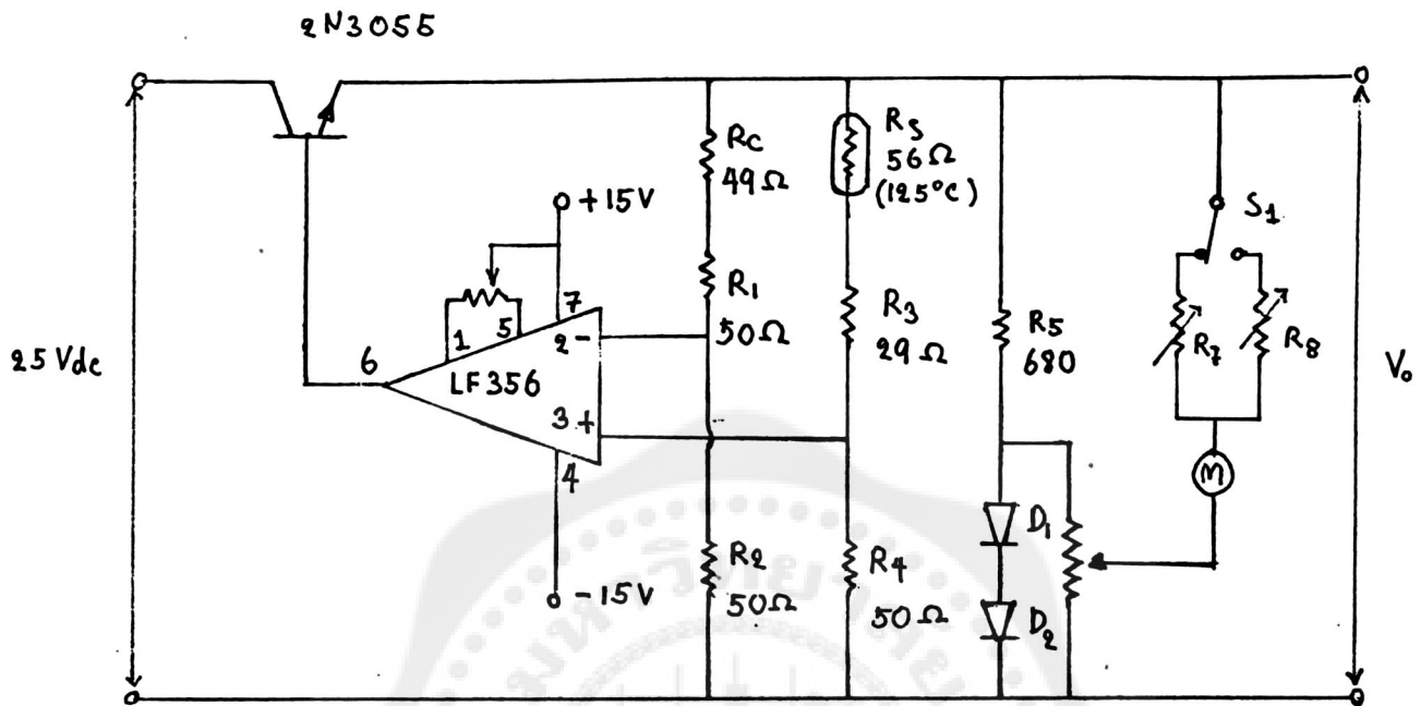
รูปที่ 2.27 วงจรวัดความดัน
