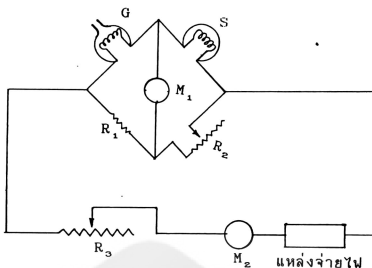
รูปที่ 1.8 วงจรวัดความต้านทานในเกจฟิรานี่
