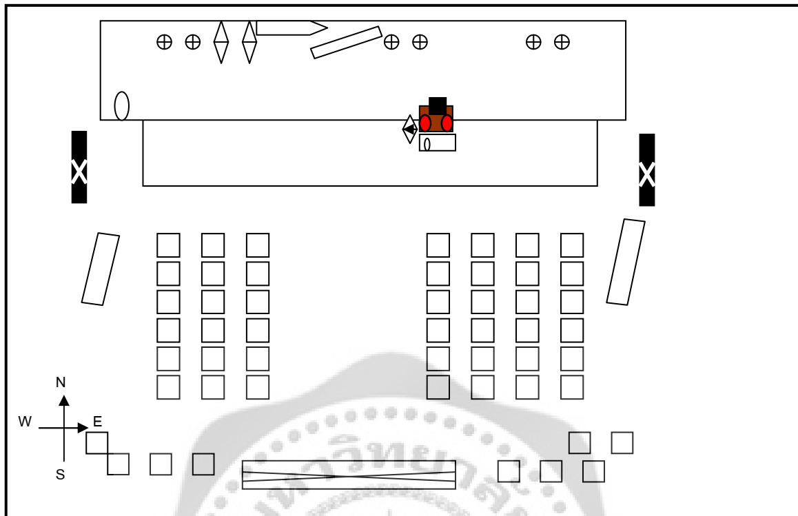
ภาพประกอบ 19 แผนผังแสดงการจัดพื้นที่ประกอบพิธี
