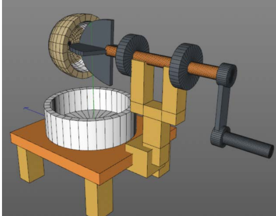
ภาพที่ ๗ เครื่องขูดมะพร้าว ๓ มิติ (ที่มา: นัทธพัชร น้อยสวัสดิ์, ๒๕๖๑)
